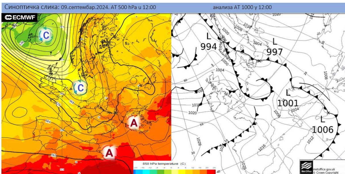
Синоптичка ситуација 09.09. у подне. (Извор: ECMWF и wetter3.de)
