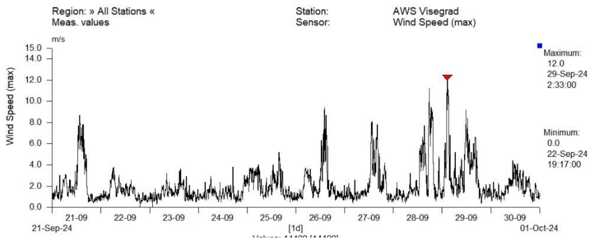
Максимални удари ветра у трећој декади септембра на АМС Вишеград
