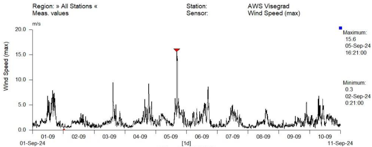
Максимални удари ветра током прве декаде на Сокоцу (горе) и Вишеграду (доле). Највеће вредности забележене су 05.09.
