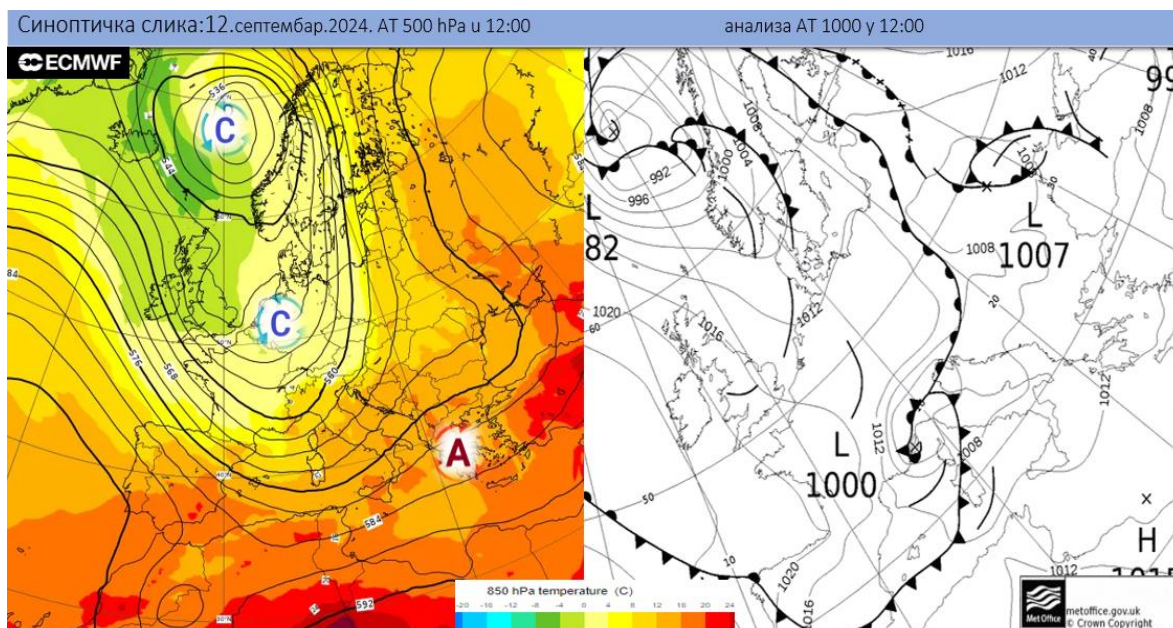
Синоптичка ситуација 12.09. у подне. (Извор: ECMWF и wetter3.de)
