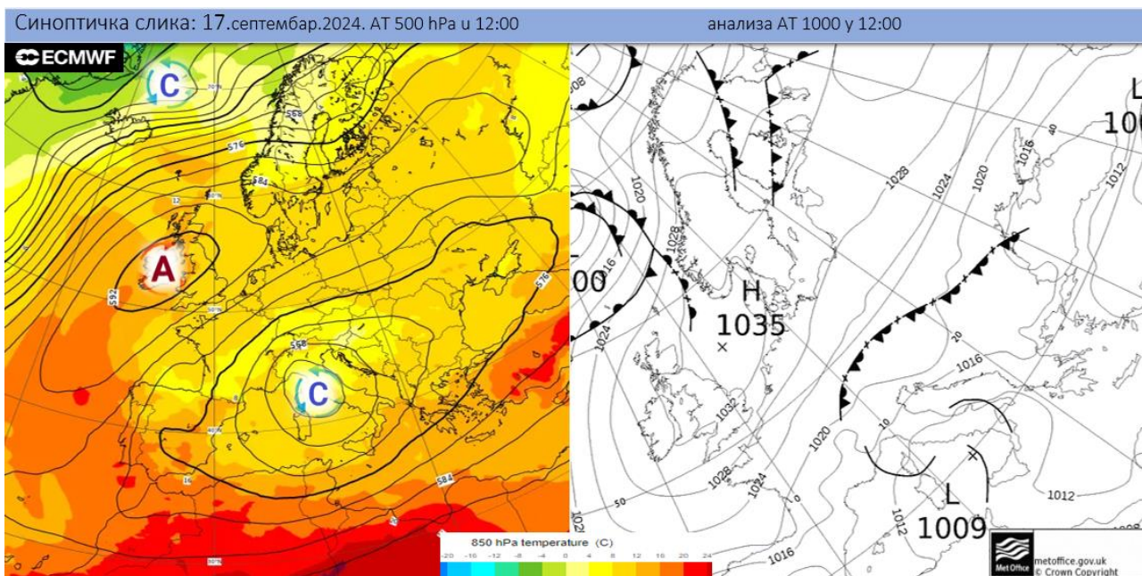
Синоптичка ситуација 17.09. у подне. (Извор: ECMWF и wetter3.de)
