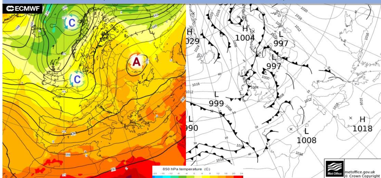
Синоптичка ситуација 24.09. у подне. (Извор: ECMWF и wetter3.de)
