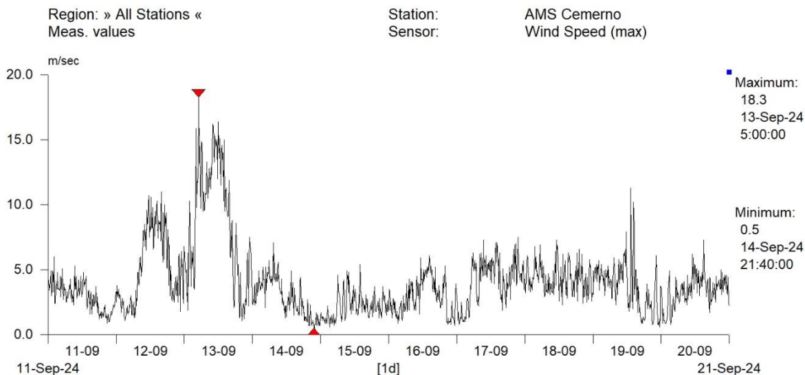
Максимални удари ветра у другој декади септембра на АМС Чемерно
