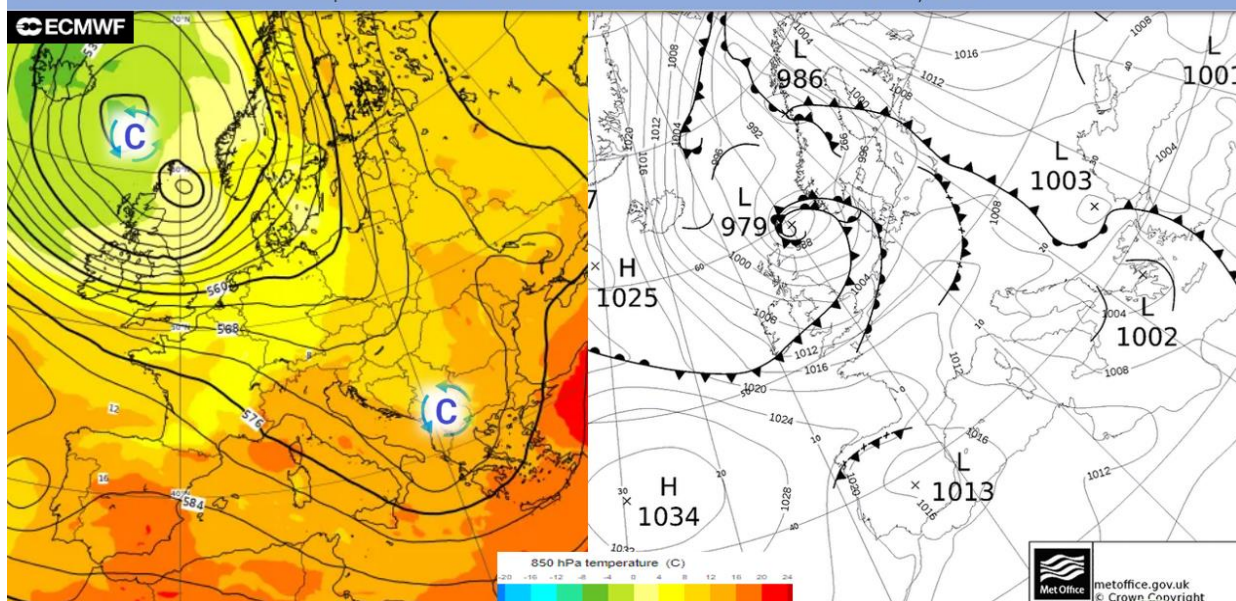
Синоптичка ситуација 10.09. у подне. (Извор: ECMWF и wetter3.de)
