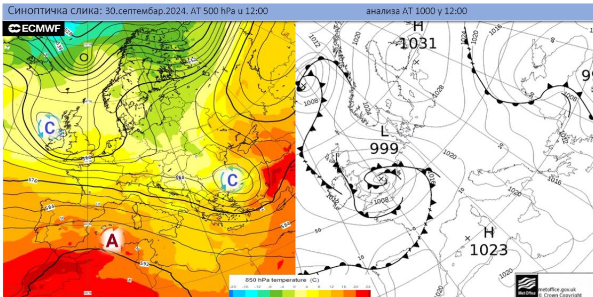
Синоптичка ситуација 30.09. у подне. (Извор: ECMWF и wetter3.de)
