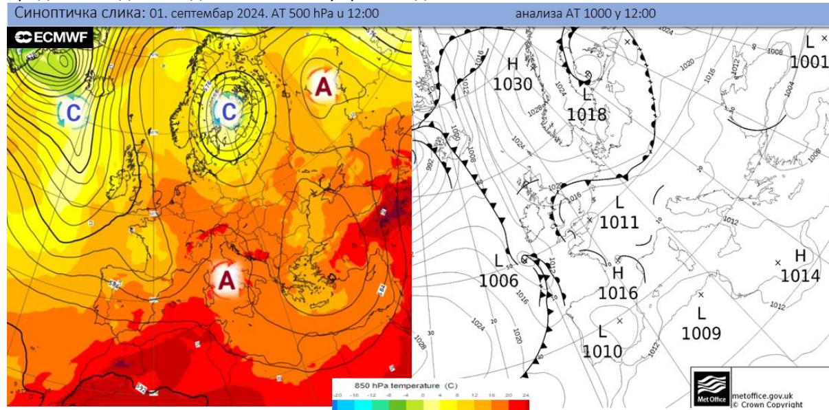
Синоптичка ситуација 01.09. у подне (извор: ECMWF и wetter3.de)
