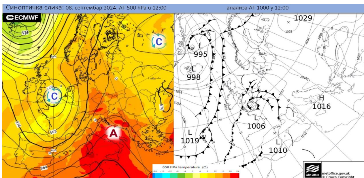
Синоптичка ситуација 08.09. у подне. (Извор: ECMWF и wetter3.de)
