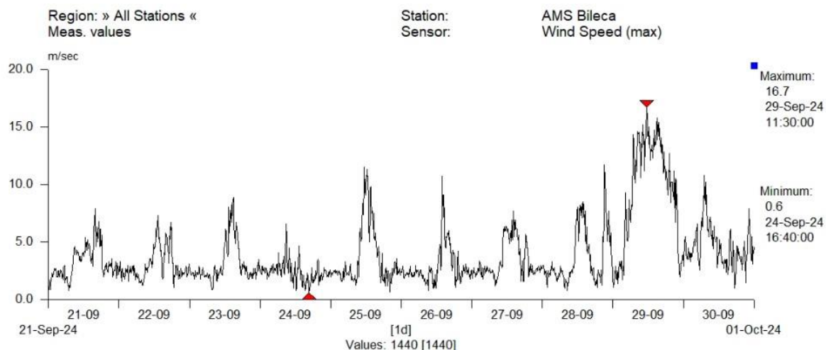
Максимални удари ветра у трећој декади септембра на АМС Билећа
