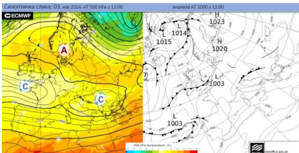
Синоптичка ситуација 03.05.2024. (извор: ECMWF и wetter3.de)
