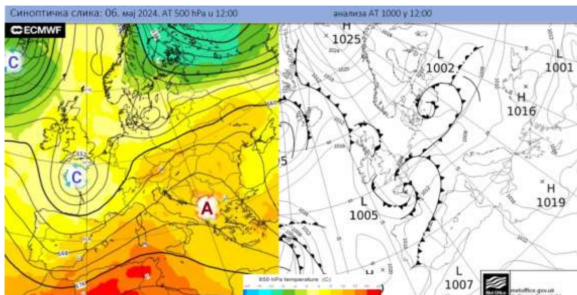
Синоптичка ситуација 06.05.2024. (извор: ECMWF и wetter3.de)
