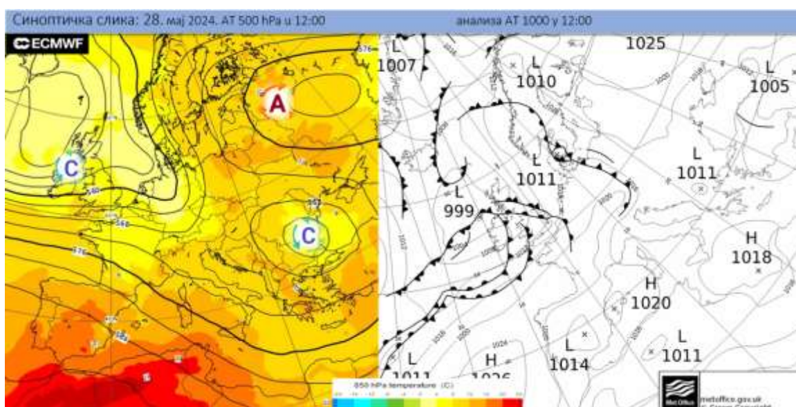
Синоптичка ситуација 28.05. (извор: ECMWF и wetter3.de)
