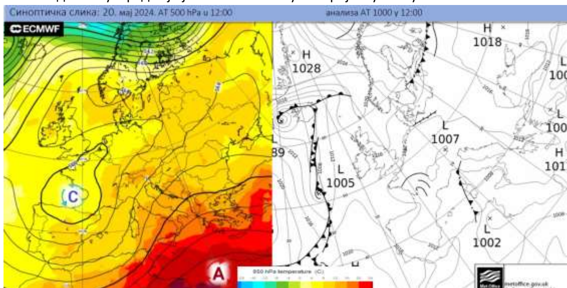
Синоптичка ситуација 20.05. (извор: ECMWF и wetter3.de)
