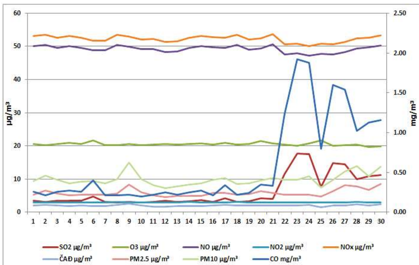
Дијаграм 4. Графички приказ просјечних имисијских дневних концетрација SO 2 ,CO, NO, NO 2 , NO x , O 3 , PM 2.5 , PM 10 и ЧАД за септембар 2026. у Бањој Луци (мјерно мјесто Борик).
