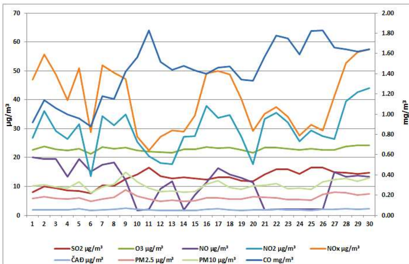
Дијаграм 3. Графички приказ просјечних имисијских дневних концентрација SO 2 , CO, NO, NO 2 , NO x , PM 2.5 , PM 10 , O 3 и ЧАД за септембар 2026. у Бањој Луци (мјерно мјесто Центар града).
