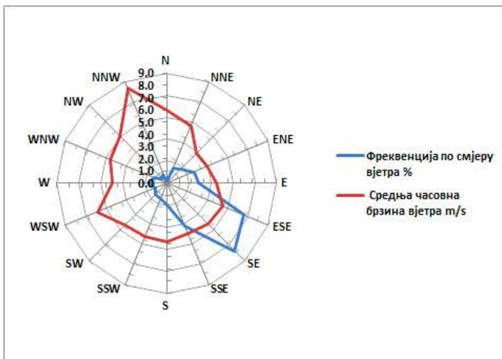
Слика 4. Приказ честине вјетра за септембар 2026. године у Требињу (мјерно мјесто круг метеоролошке станице у Требињу)
