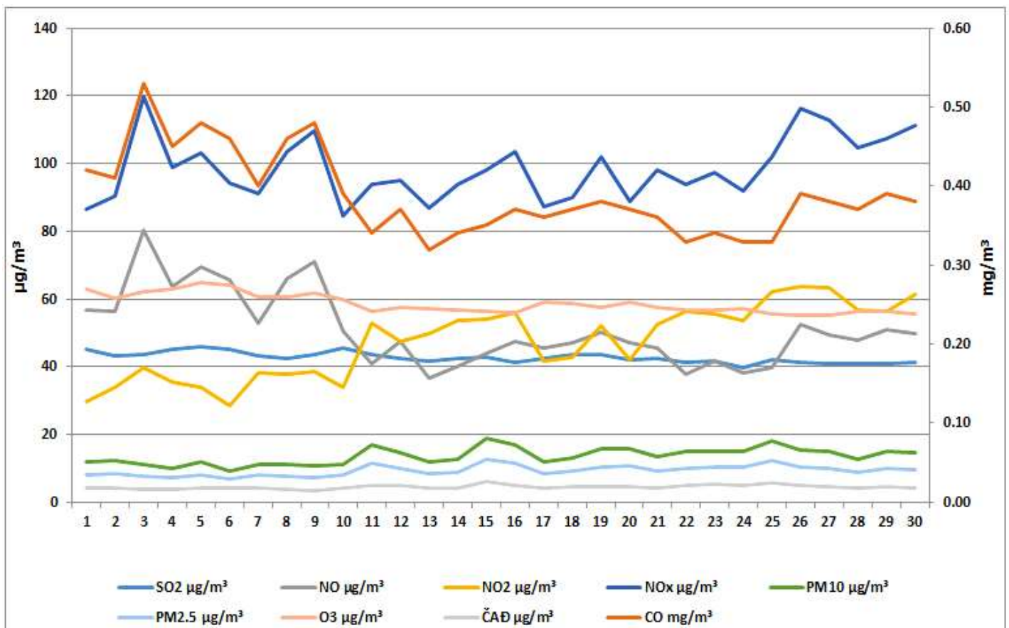
Дијаграм 7. Графички приказ просјечних имисијских дневних концентрација SO 2 , CO, NO, NO 2 , NO x , O 3 , ČАД, PM 2.5 и PM 10 за септембар 2026. у Бијељини (мјерно мјесто Топлана).
