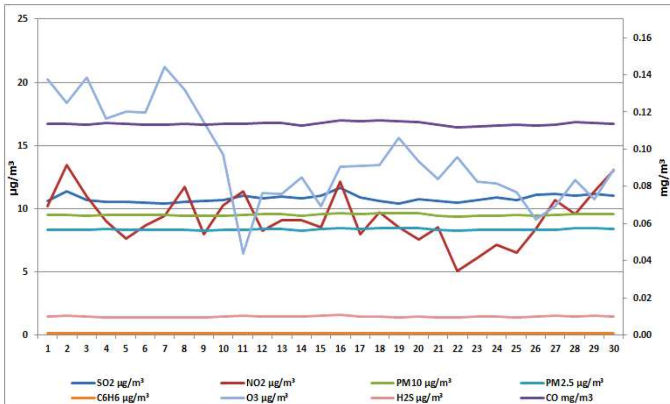
Дијаграм 9. Графички приказ просјечних имисијских дневних концентрација SO 2 , CO, O 3 , C 6 H 6 , H 2 S, NO 2 , PM 2.5 , и PM 10 честица засептембар 2026. у Броду (мјерно мјесто Рафинерија нафте Брод а.д.)
