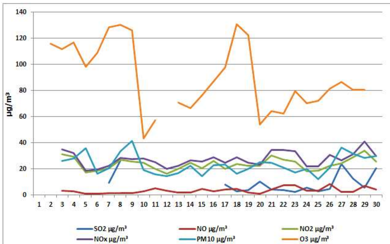
Дијаграм 11. Графички приказ просјечних имисијских дневних концентрација NO, NO 2 , NO x , PM 10 , O 3 и SO 2 за септембар 2026. у Добоју (мјерно мјесто круг метеоролошке станице у Добоју)
