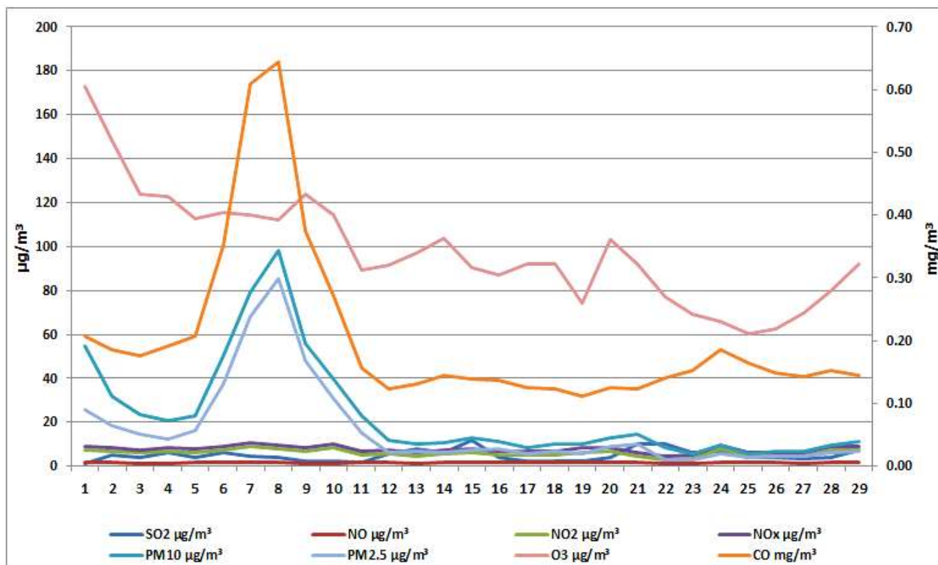
Дијаграм 10. Графички приказ просјечних имисијских дневних концентрација SO 2 , NO, NO 2 , NO x , CO, PM 10 , O 3 и PM 2.5 честица за септембар 2026. у Требињу (мјерно мјесто круг метеоролошке станице у Требињу)
