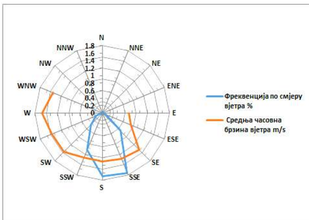
Слика 2. Приказ честине вјетра за септембар 2026. у Гацку (мјерном мјесту круг ОШ „Свети Сава“).
