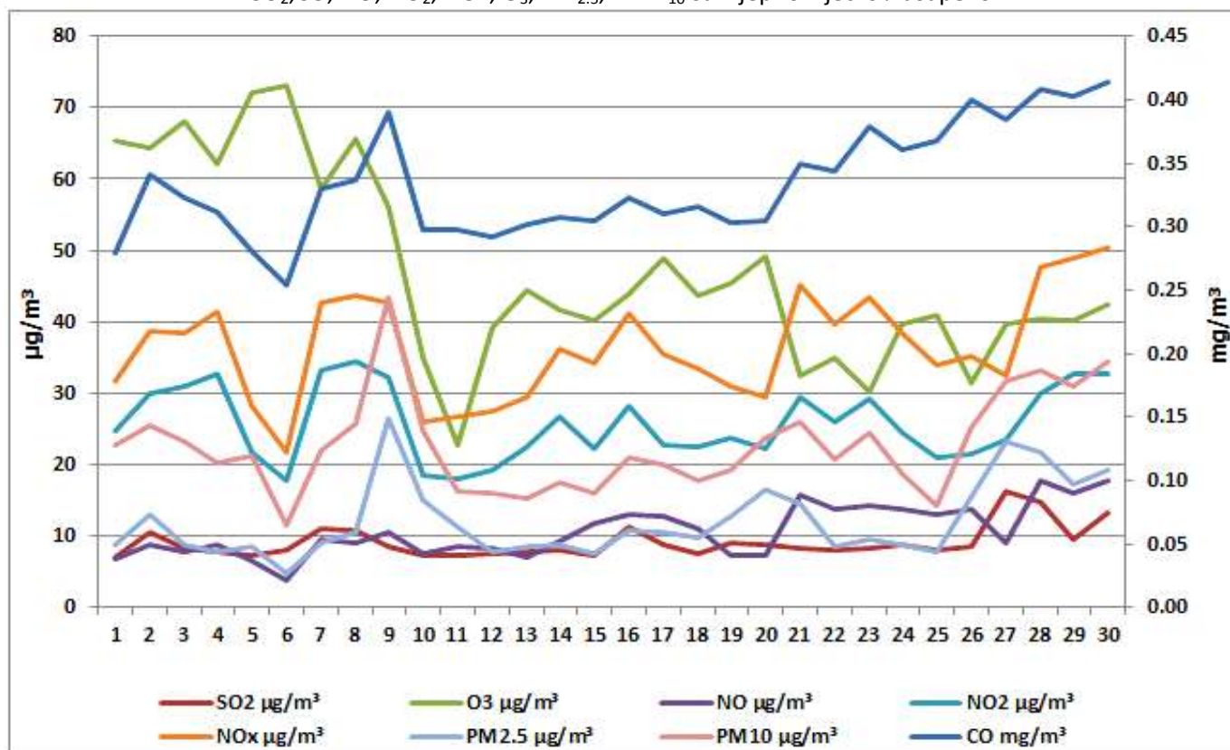
Дијаграм 1. Графички приказ просјечних имисијских дневних концентрација SO 2 , CO, NO, NO 2 , NO x , O 3 , PM 2.5 , и PM 10 за септембар 2026 у Бањој Луци (мјерно мјесто Лазарево).
