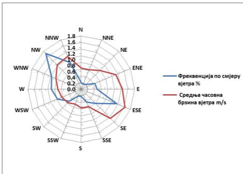
Слика 3. Приказ честине вјетра за септембар 2026. године у Броду (мјерно мјесто Рафинерија нафте Брод а.д.)
