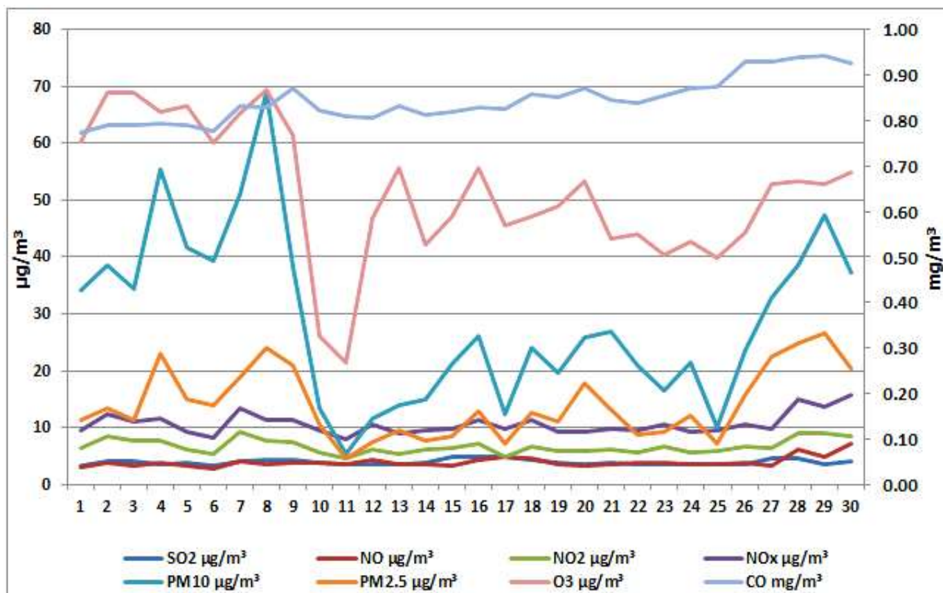
Дијаграм 5. Графички приказ просјечних имисијских дневних концентрација SO 2 , NO, NO 2 , NO x , PM 2.5 , PM 10 , CO и O 3 за септембар 2026. у Приједору (мјерно мјесто круг метеоролошке станице у Приједору)
