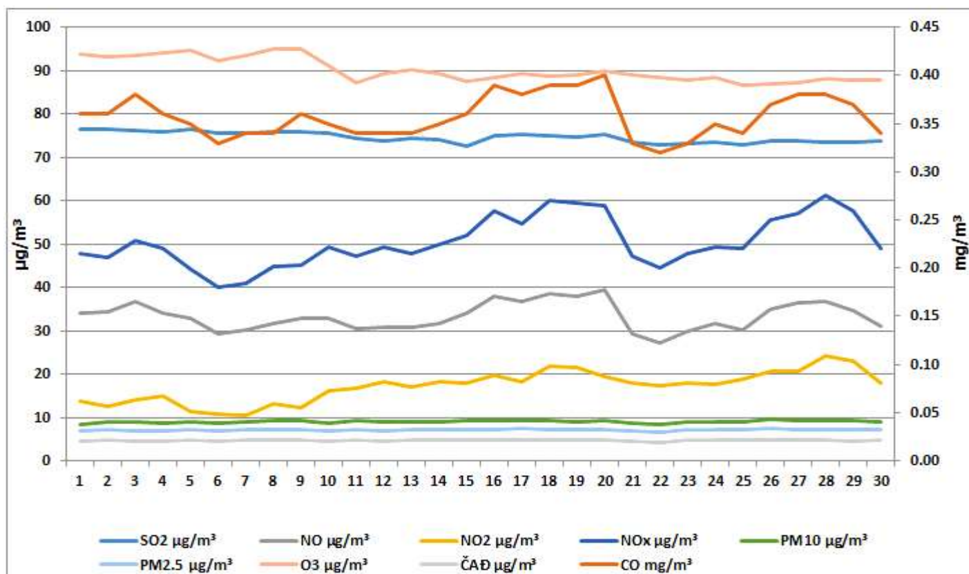
Дијаграм 6. Графички приказ просјечних имисијских дневних концентрација SO 2 , CO, NO, NO 2 , NO x , O 3 , ČАД, PM 2.5 и PM 10 за септембар 2026. у Бијељини (мјерно мјесто Центар града)
