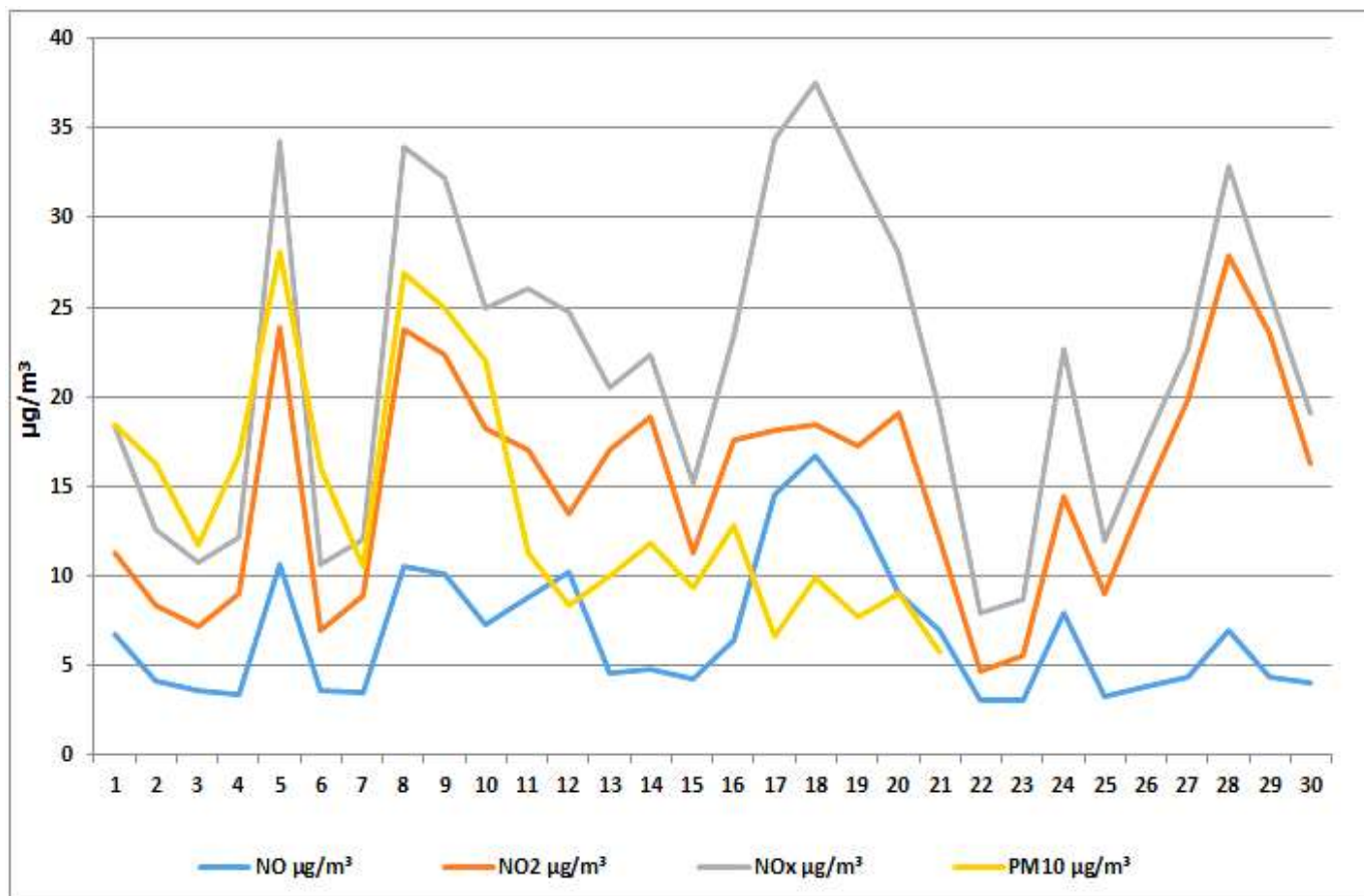
Дијаграм 8. Графички приказ просјечних имисијских дневних концентрација PM_{10} , NO , NO_2 и NOx за септембар 2026. у Гацку (мјерном мјесту круг ОШ „Свети Сава“).
