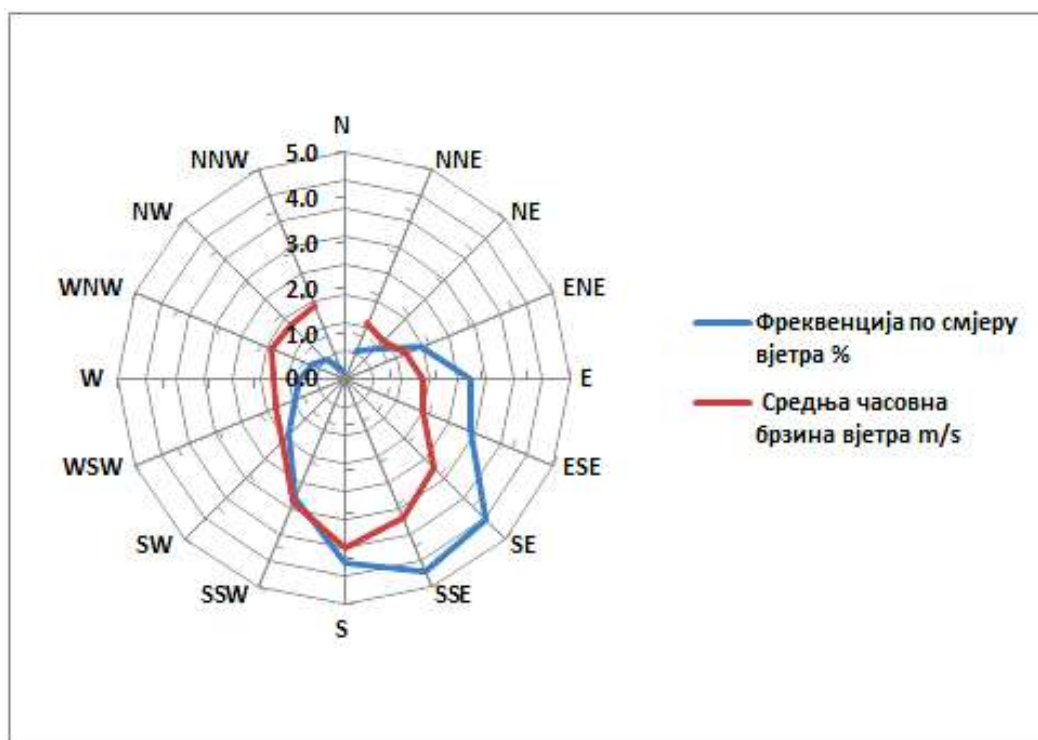
Слика 1. Приказ честине вјетра за септембар 2026. У Бања Луци (мјерно мјесто Лазарево).
