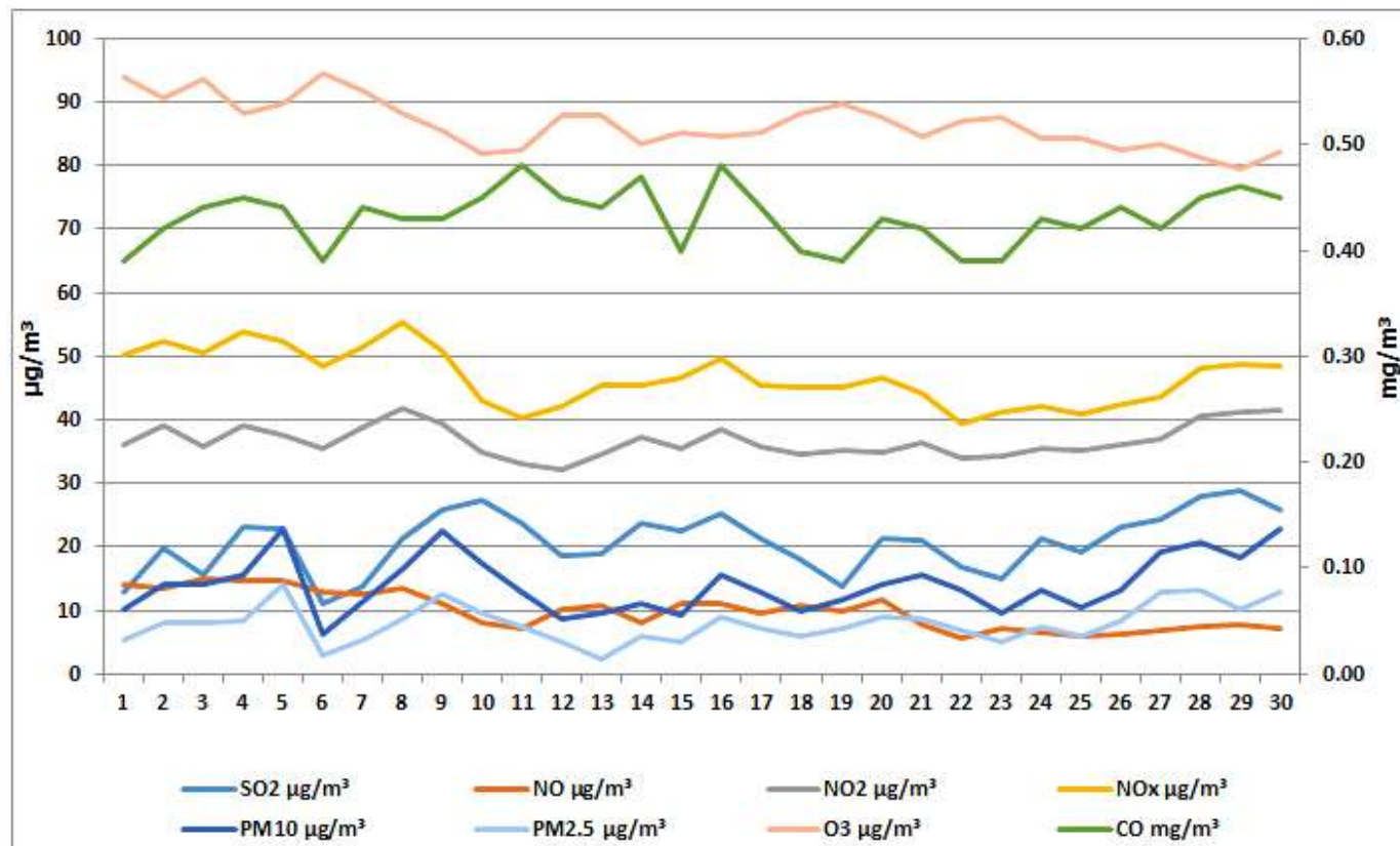
Дијаграм 12. Графички приказ просјечних имисијских дневних концентрација SO 2 , NO, NO 2 , NO x , O 3 , PM 10 , PM 2.5 и CO честица за септембар 2026. у Градишци на мјерном мјесту „Културни центар“.
