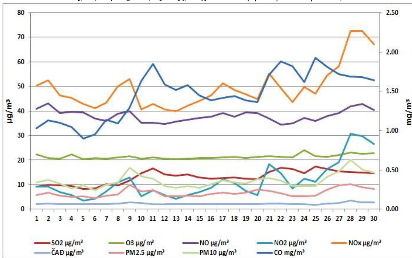
Дијаграм 2. Графички приказ просјечних имисијских дневних концентрација SO 2 ,CO, NO, NO 2 , NO x , O 3 , PM 2.5 , PM 10 и ЧАД за септембар 2026. у Бањој Луци (мјерно мјесто Паприковац).
