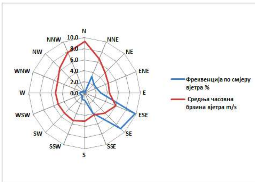
Слика 4. Приказ честине вјетра за август 2026. године у Требињу (мјерно мјесто круг метеоролошке станице у Требињу)
