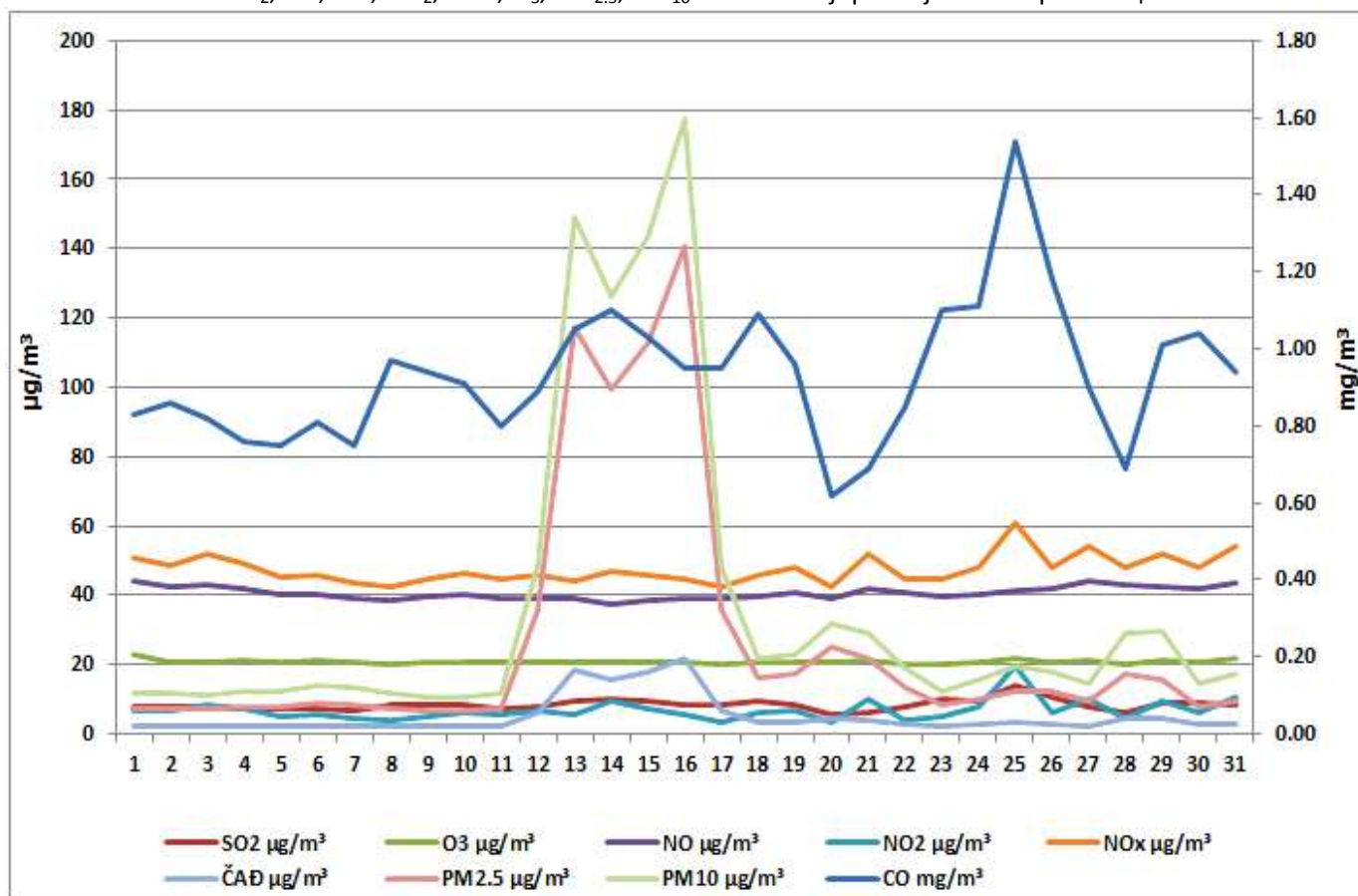
Дијаграм 2. Графички приказ просјечних имисијских дневних концентрација SO 2 , CO, NO, NO 2 , NO x , O 3 , PM 2.5 , PM 10 и ЧАД за август 2026. у Бањој Луци (мјерно мјесто Паприковац).
