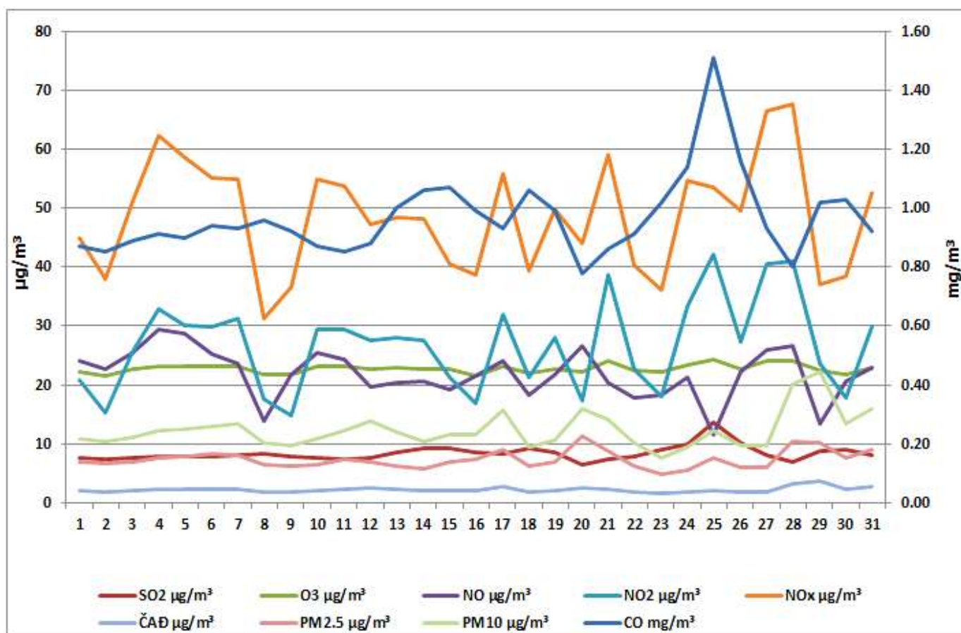
Дијаграм 3. Графички приказ просјечних имисијских дневних концентрација SO 2 , CO, NO, NO 2 , NO x , PM 2.5 , PM 10 , O 3 и ČАД за август 2026. у Бањој Луци (мјерно мјесто Центар града).
