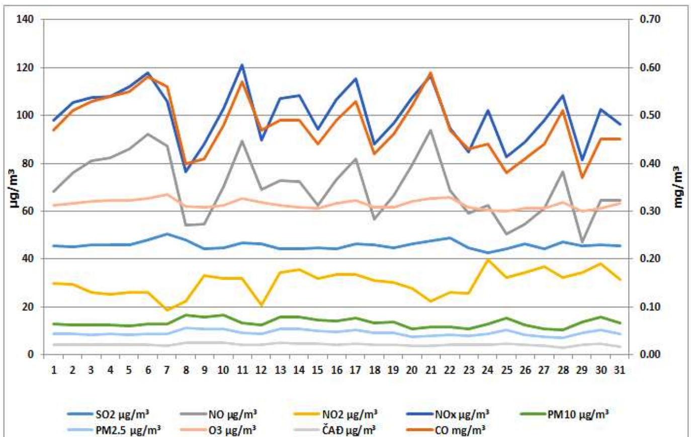
Дијаграм 7. Графички приказ просјечних имисијских дневних SO 2 , CO, NO, NO 2 , NO x , O 3 , ЧАД, PM 2.5 и PM 10 за август 2026. у Бијељини (мјерно мјесто Топлана).
