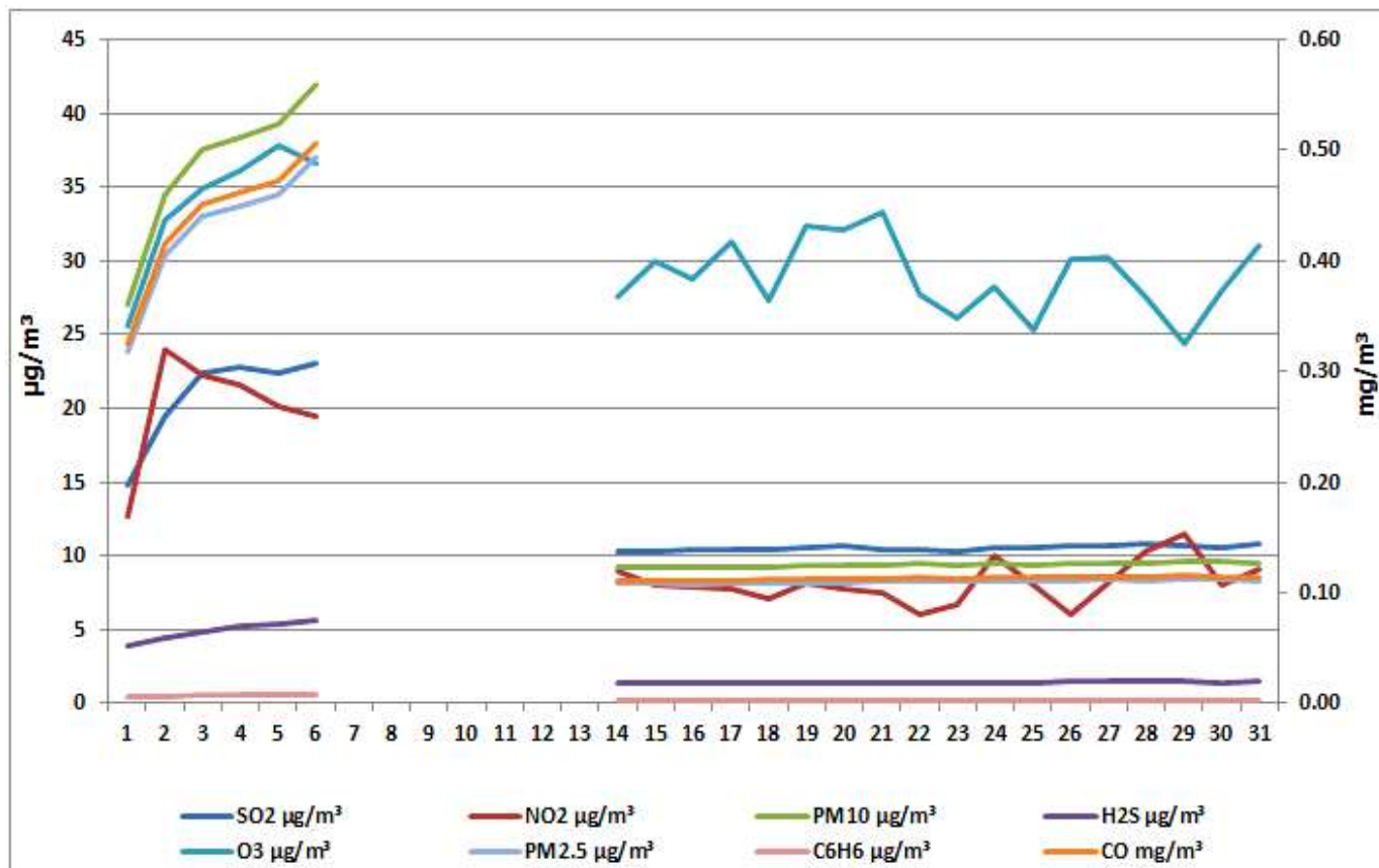
Дијаграм 9. Графички приказ просјечних имисијских дневних концентрација SO 2 , CO, O 3 , C 6 H 6 , H 2 S, NO 2 , PM 2.5 , и PM 10 честица за август 2026. у Броду (мјерно мјесто Рафинерија нафте Брод а.д.)
