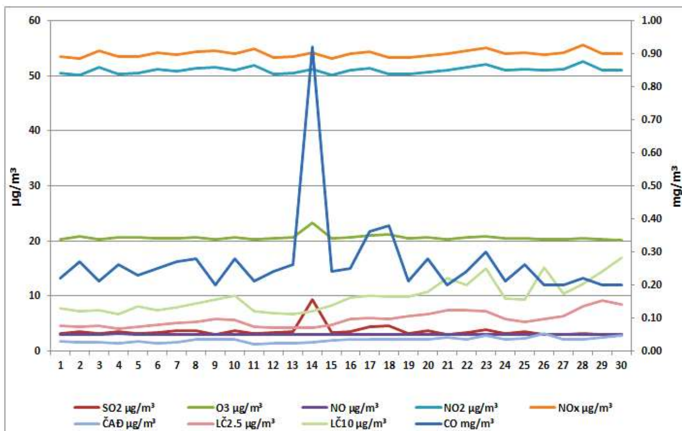
Дијаграм 4. Графички приказ просјечних имисијских дневних концентратија SO 2 ,CO, NO, NO 2 , NO x , O 3 , PM 2.5 , PM 10 и ЧАД за јун 2026. у Бањој Луци (мјерно мјесто Борик).
