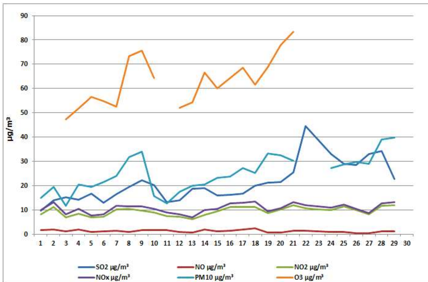
Дијаграм 11. Графички приказ просјечних имисијских дневних концентрација NO, NO 2 , NO x , PM 10 , O 3 и SO 2 за јун 2026. у Добоју (мјерно мјесто круг метеоролошке станице у Добоју)
