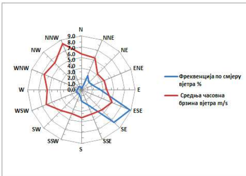
Слика 4. Приказ честине вјетра за јун 2026. године у Требињу (мјерно мјесто круг метеоролошке станице у Требињу)
