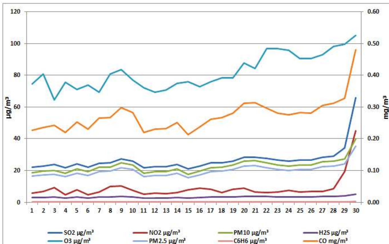
Дијаграм 9. Графички приказ просјечних имисијских дневних концентрација SO 2 , CO, O 3 , C 6 H 6 , H 2 S, NO 2 , PM 2.5 , и PM 10 честица за јун 2026. у Броду (мјерно мјесто Рафинерија нафте Брод а.д.)
