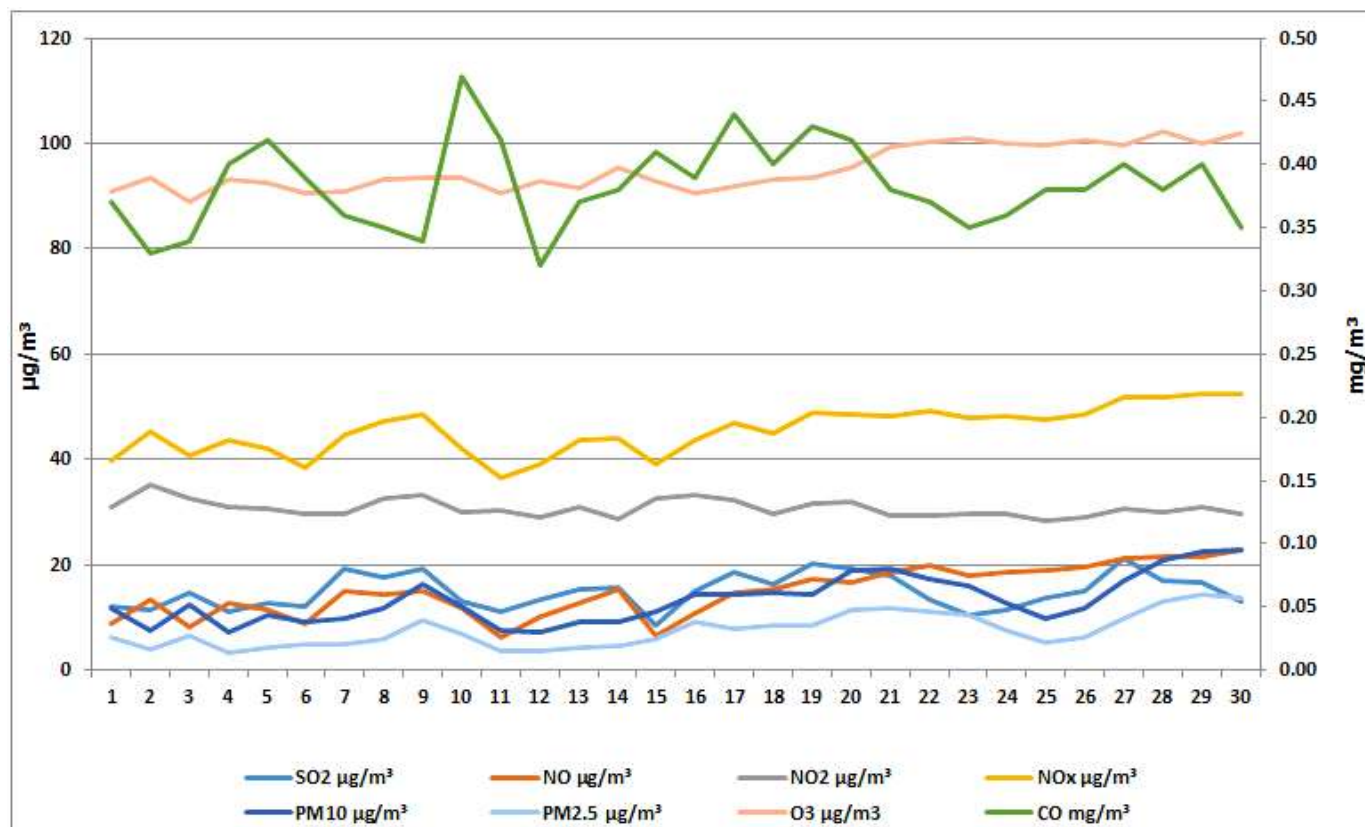
Дијаграм 12. Графички приказ просјечних имисијских дневних концентрација SO 2 , NO, NO 2 , NO x , O 3 , PM 10 , PM 2.5 и CO честица за јун 2026. у Градишци на мјерном мјесту „Културни центар“.
