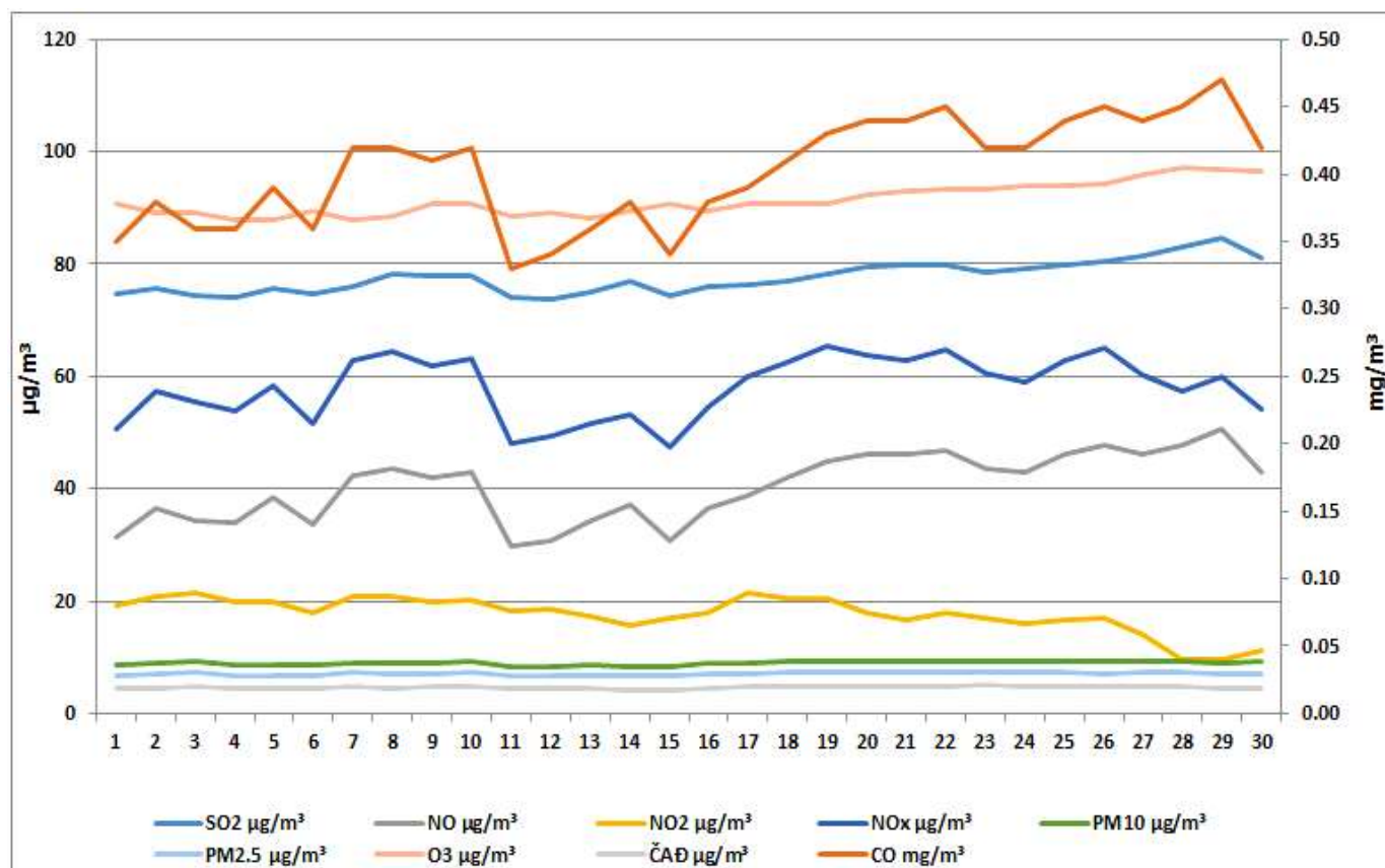
Дијаграм 6. Графички приказ просјечних имисијских дневних SO 2 , CO, NO, NO 2 , NO x , O 3 , ČАД, PM 2.5 и PM 10 за јун 2026. у Бијељини (мјерно мјесто Центар града)
