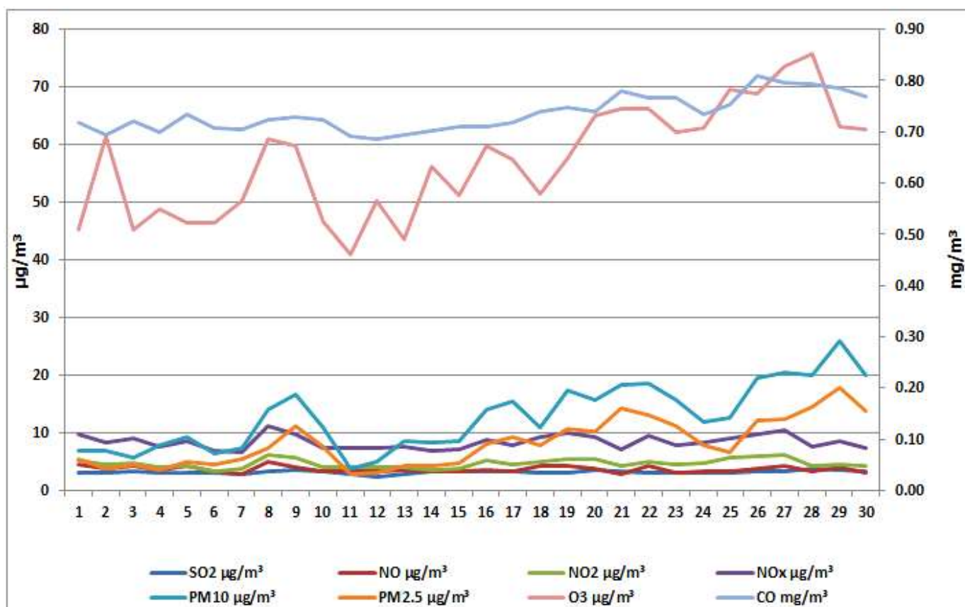
Дијаграм 5. Графички приказ просјечних имисијских дневних концентрација SO 2 , NO, NO 2 , NO x , PM 2.5 , PM 10 , CO и O 3 за јун 2026. у Приједору (мјерно мјесто круг метеоролошке станице у Приједору)
