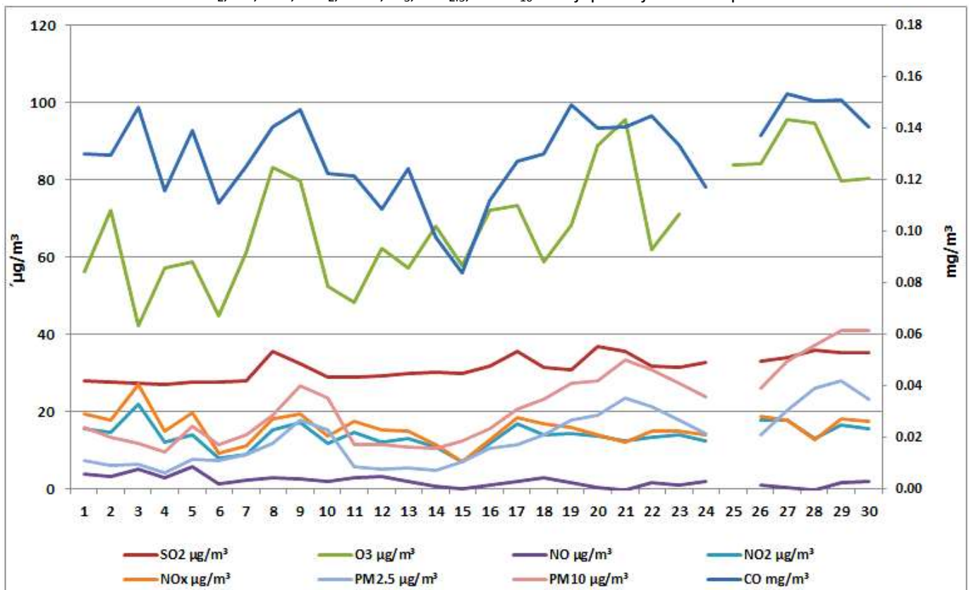
Дијаграм 1. Графички приказ просјечних имисијских дневних концентратија SO 2 , CO, NO, NO 2 , NO x , O 3 , PM 2.5 и PM 10 за јун 2026 у Бањој Луци (мјерно мјесто Лазарево).
