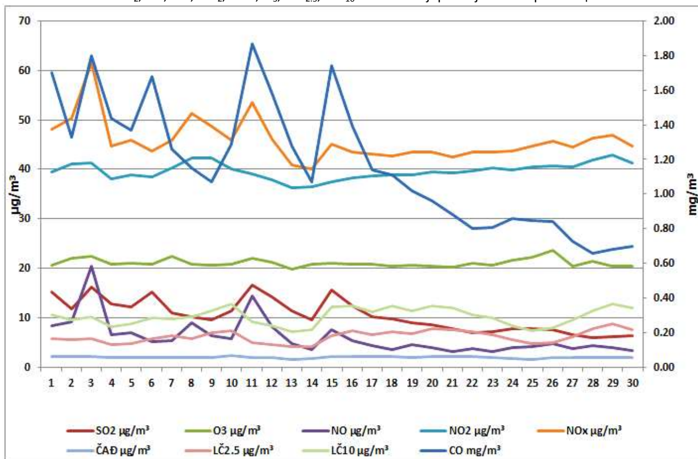
Дијаграм 2. Графички приказ просјечних имисијских дневних концентрација SO 2 , CO, NO, NO 2 , NO x , O 3 , PM 2.5 , PM 10 и ЧАД за јун 2026. у Бањој Луци (мјерно мјесто Паприковац).
