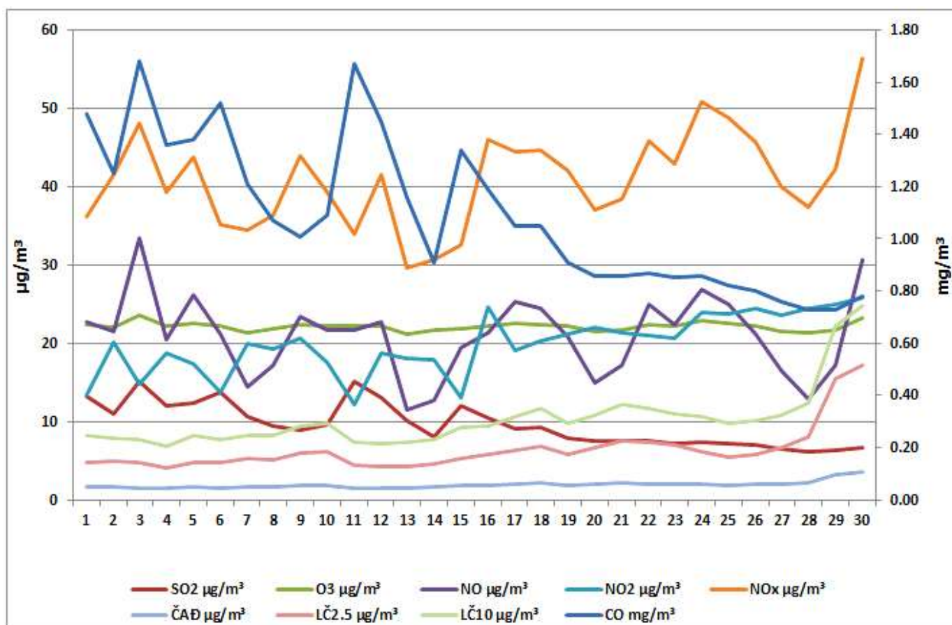
Дијаграм 3. Графички приказ просјечних имисијских дневних концентрација SO 2 , CO, NO, NO 2 , NO x , PM 2.5 , PM 10 , O 3 и ČАД за јун 2026. у Бањој Луци (мјерно мјесто Центар града).
