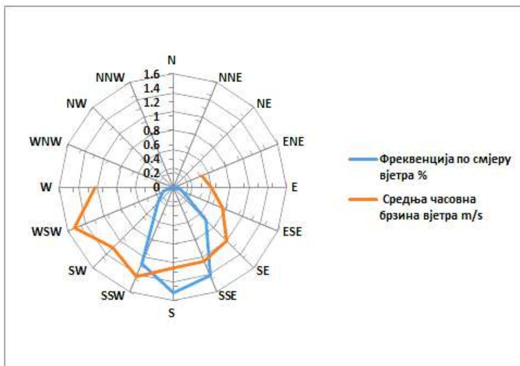
Слика 2. Приказ честине вјетра за јун 2026. у Гацку (мјерном мјесту круг ОШ „Свети Сава“).
