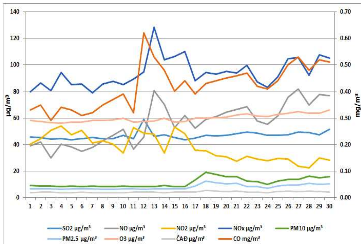
Дијаграм 7. Графички приказ просјечних имисијских дневних SO 2 , CO, NO, NO 2 , NO x , O 3 , ЧАД, PM 2.5 и PM 10 за јун 2026. у Бијељини (мјерно мјесто Топлана).
