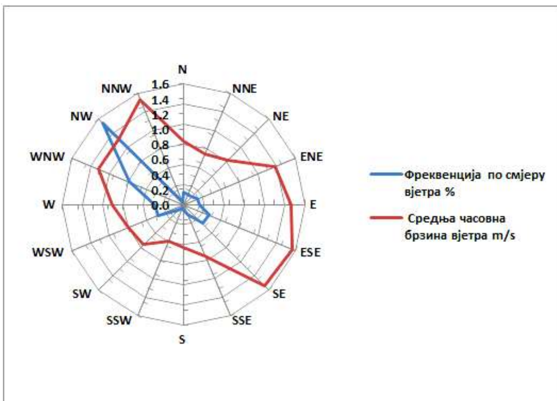
Слика 3. Приказ честине вјетра за јун 2026. године у Броду (мјерно мјесто Рафинерија нафте Брод а.д.)
