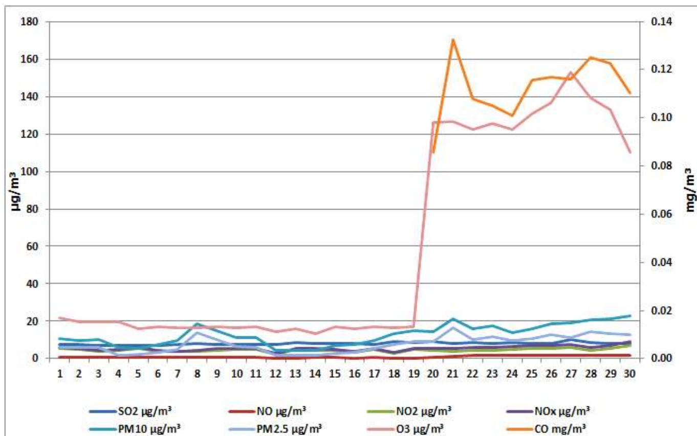
Дијаграм 10. Графички приказ просјечних имисијских дневних концентрација SO 2 , NO, NO 2 , NO x , CO, PM 10 , O 3 и PM 2.5 честица за јун 2026. у Требињу (мјерно мјесто круг метеоролошке станице у Требињу)
