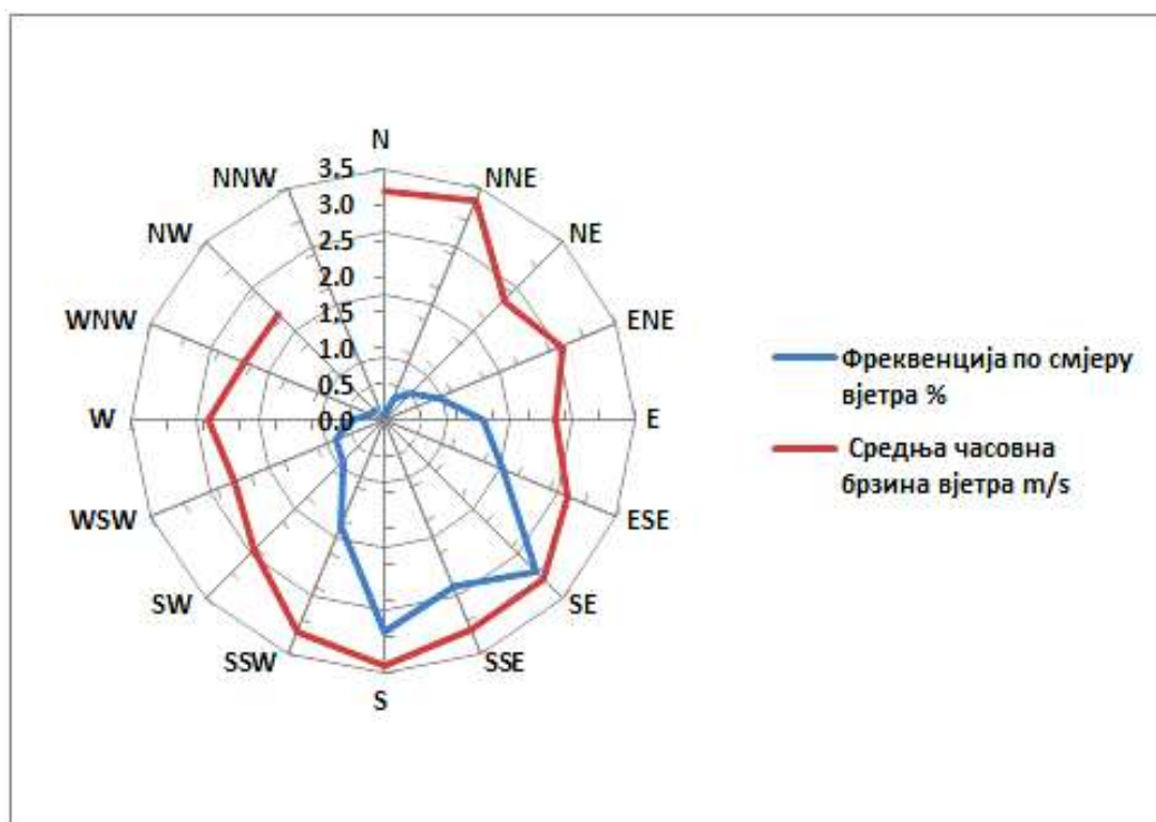
Слика 1. Приказ честине вјетра за јун 2026. У Бања Луци (мјерно мјесто Лазарево).
