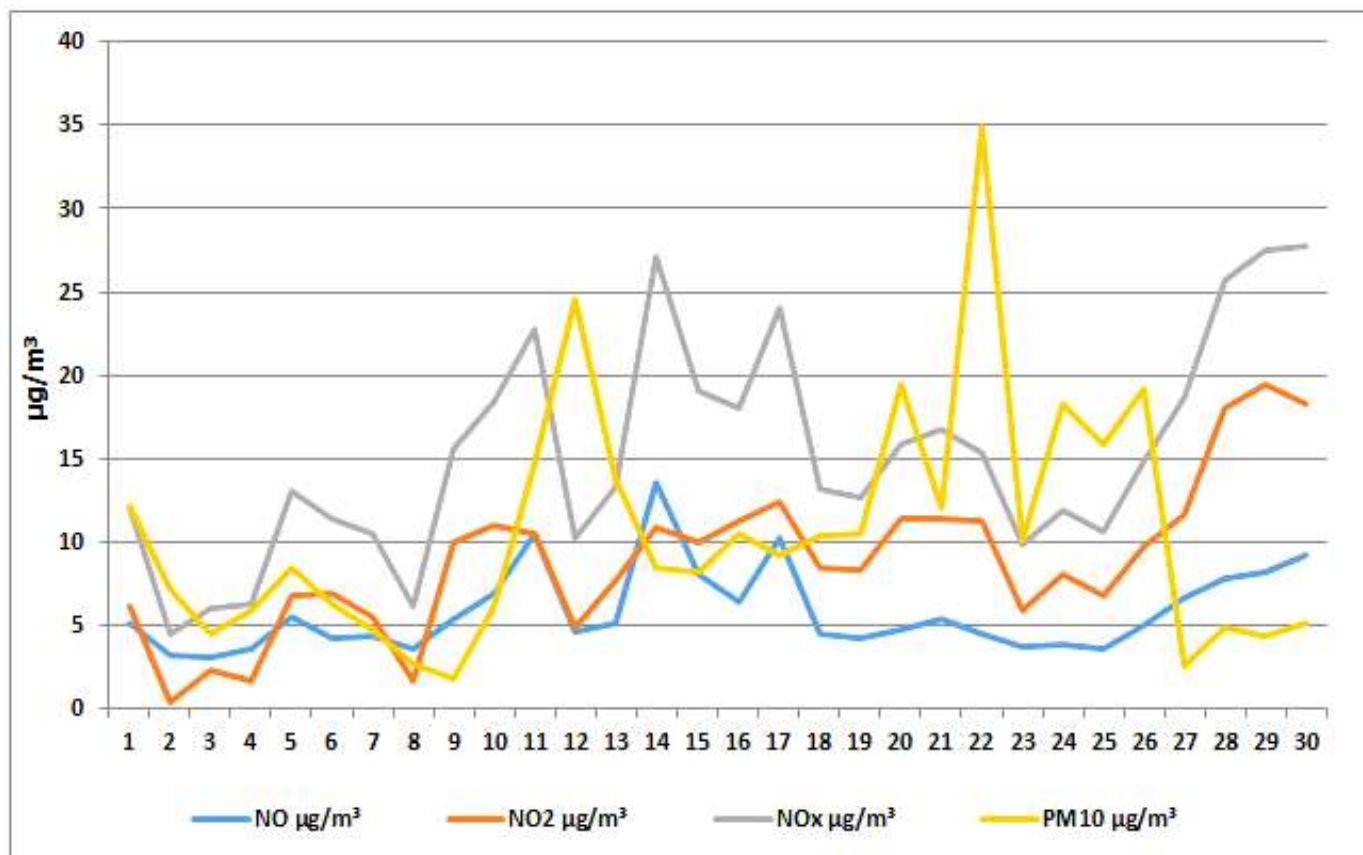
Дијаграм 8. Графички приказ просјечних имисијских дневних концентрација PM_{10} , NO , NO_2 и NO_x за јун 2026. у Гацку (мјерном мјесту круг ОШ „Свети Сава“).
