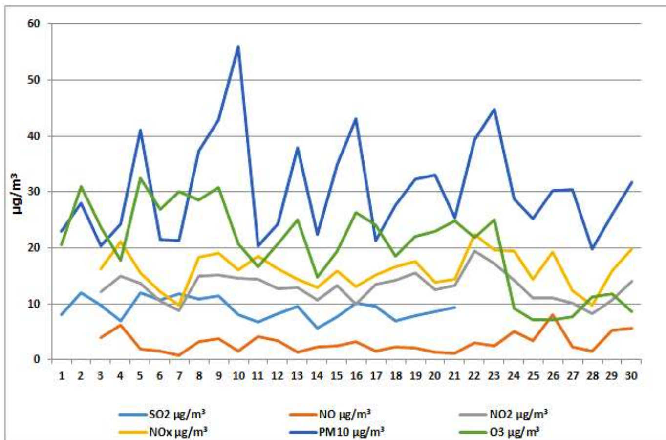
Дијаграм 11. Графички приказ просјечних имисијских дневних концентрација NO, NO 2 , NO x , PM 10 , O 3 и SO 2 за септембар 2025. у Добоју (мјерно мјесто круг метеоролошке станице у Добоју)
