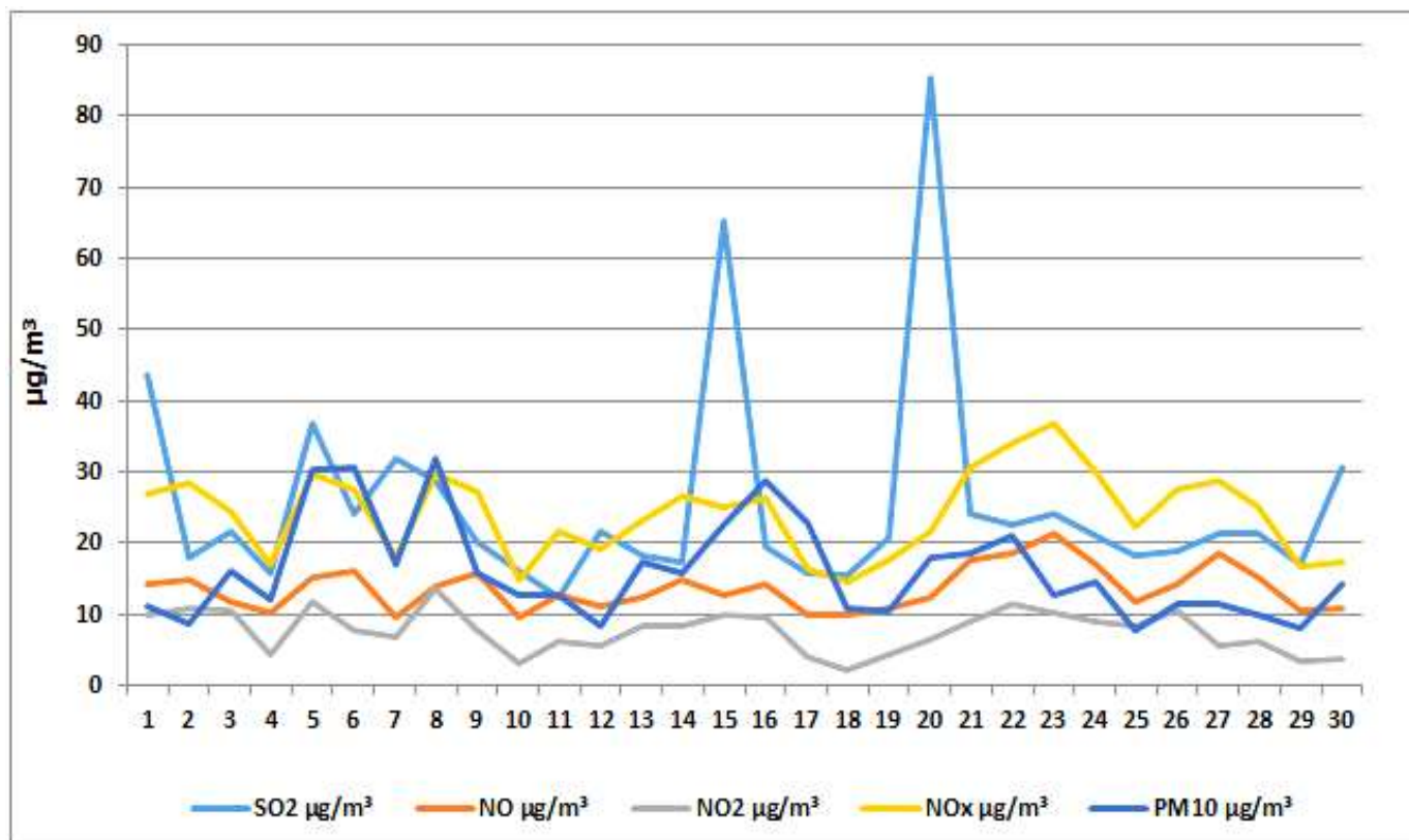
Дијаграм 7. Графички приказ просјечних имисијских дневних концентрација \text{SO}_2 , \text{PM}_{10} , \text{NO} , \text{NO}_2 и \text{NOx} за септембар 2025. у Гацку (мјерном мјесту круг ОШ „Свети Сава“).
