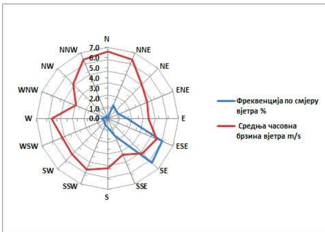
Слика 4. Приказ честине вјетра за септембар 2025. године у Требињу (мјерно мјесто круг метеоролошке станице у Требињу)
