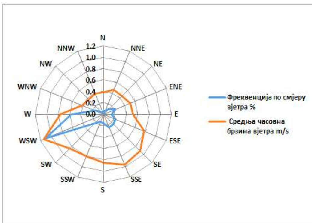
Слика 5. Приказ честине вјетра за септембар 2025. године у Добоју (мјерно мјесто круг метеоролошке станице у Добоју)
