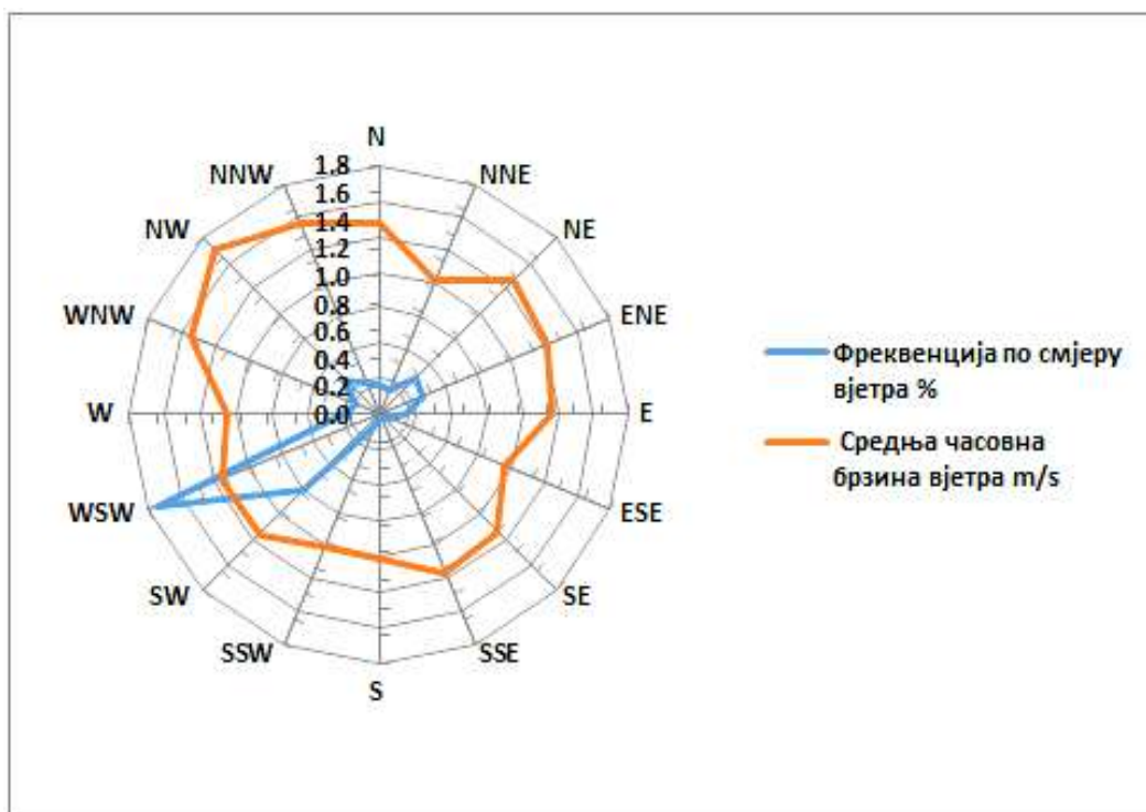
Слика 2. Приказ честине вјетра за септембар 2025. у Угљевику (мјерном мјесту круг Т.Е.Угљевик).
