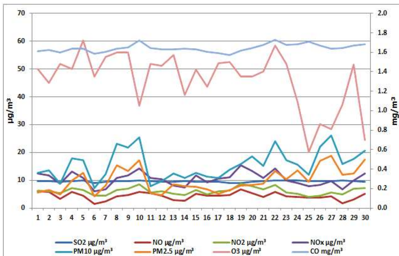
Дијаграм 5. Графички приказ просјечних имисијских дневних концентрација SO 2 , NO, NO 2 , NO x , PM 2.5 , PM 10 , CO и O 3 за септембар 2025. у Приједору (мјерно мјесто круг метеоролошке станице у Приједору)
