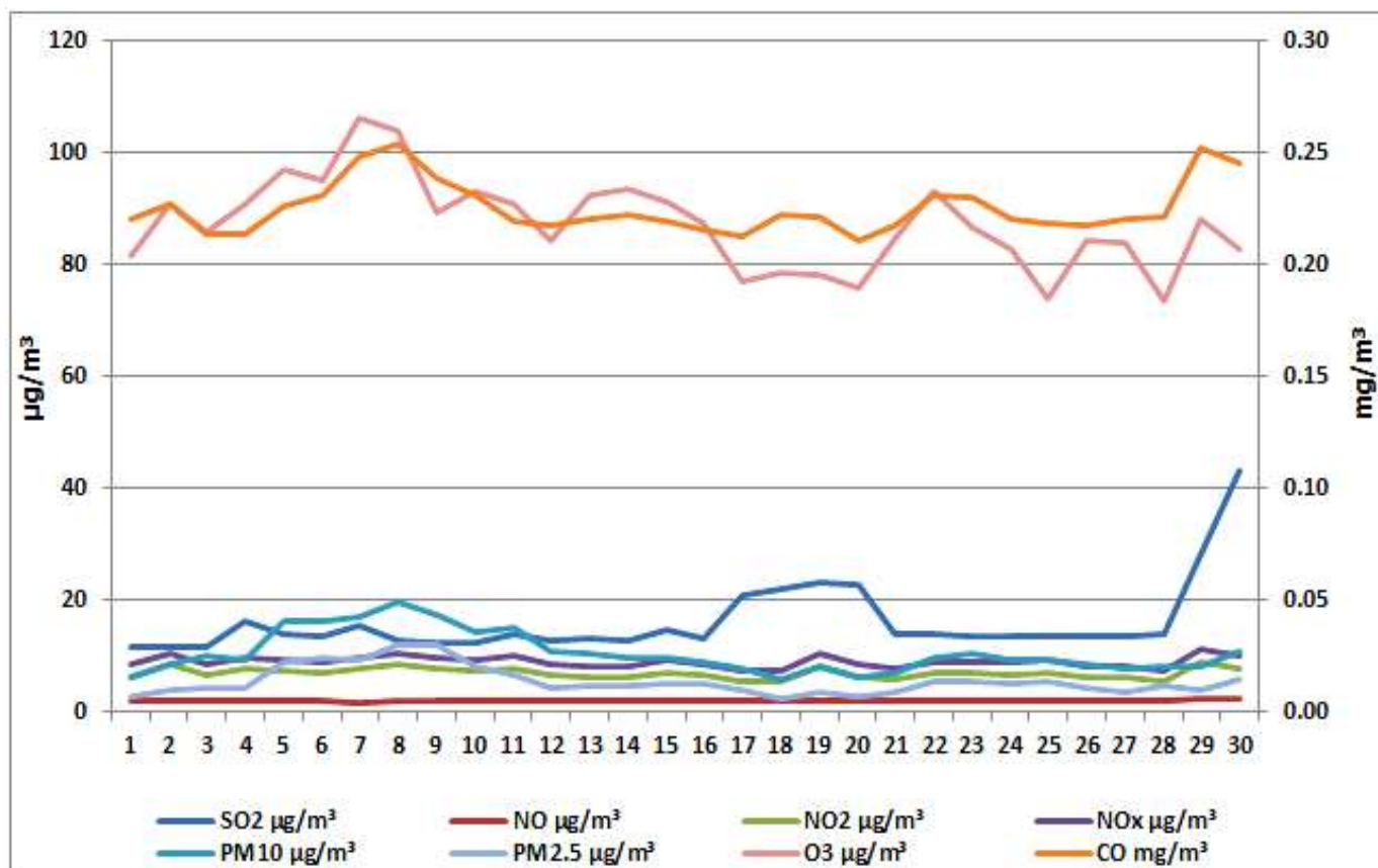
Дијаграм 10. Графички приказ просјечних имисијских дневних концентрација SO 2 , NO, NO 2 , NO x , CO, PM 10 , O 3 и PM 2.5 честица за септембар 2025. у Требињу (мјерно мјесто круг метеоролошке станице у Требињу)
