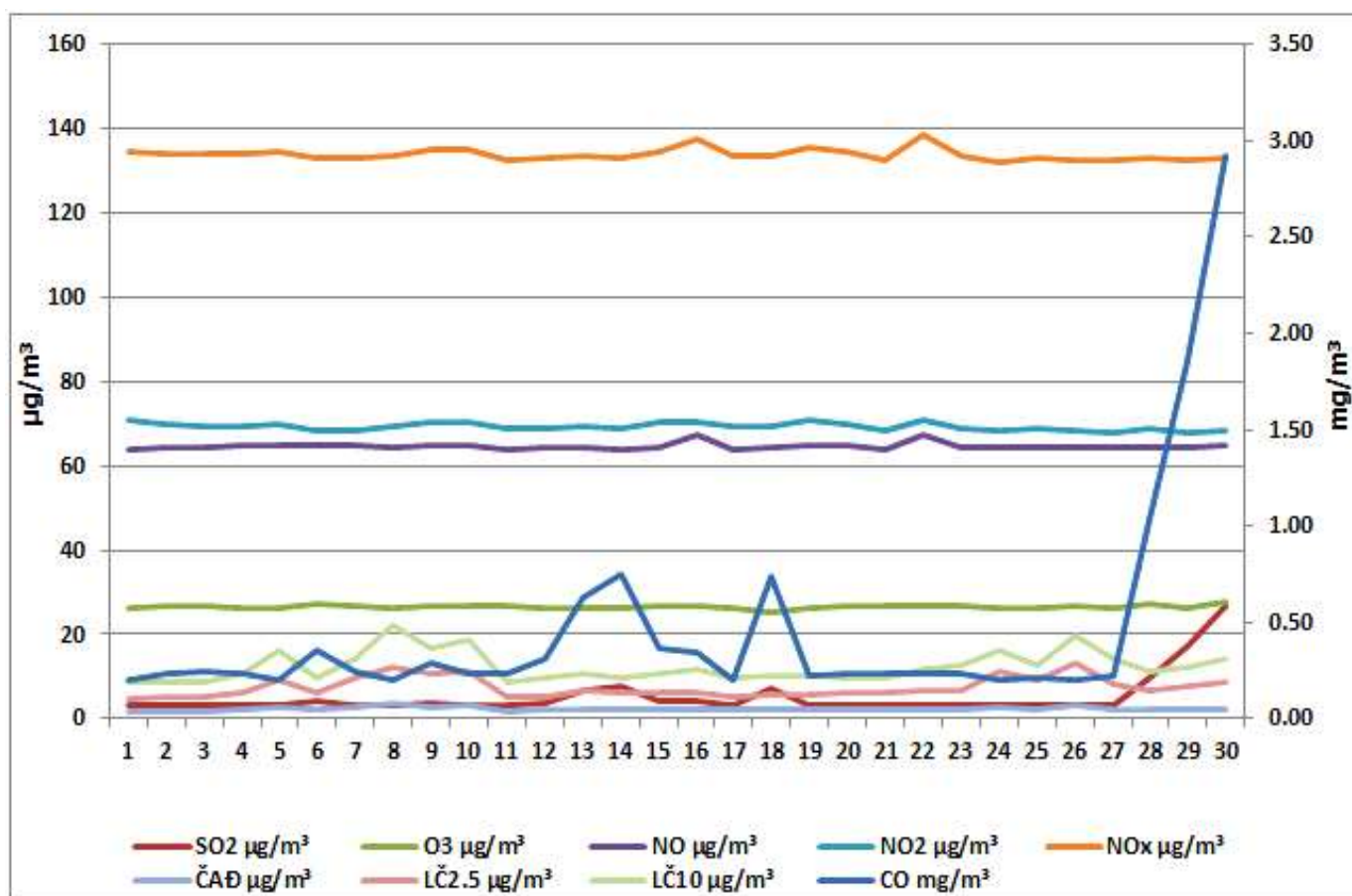
Дијаграм 4. Графички приказ просјечних имисијских дневних концентрација SO 2 ,CO, NO, NO 2 , NO x , O 3 , PM 2.5 , PM 10 и ЧАД за септембар 2025. у Бањој Луци (мјерно мјесто Борик)
