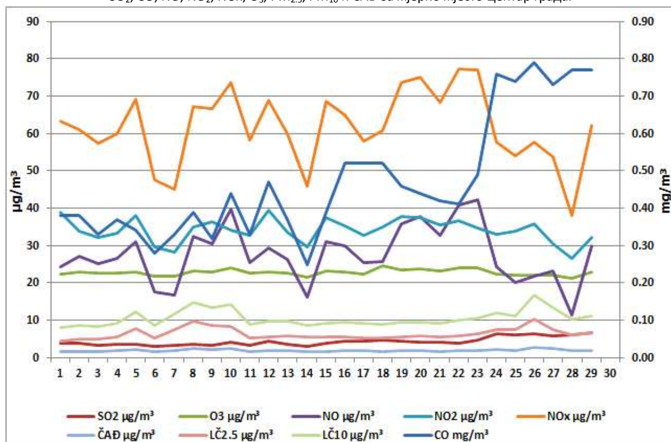
Дијаграм 3. Графички приказ просјечних имисијских дневних концентратија SO 2 , CO, NO, NO 2 , NO x , PM 2.5 , PM 10 , O 3 и ЧАД за септембар 2025. у Бањој Луци (мјерно мјесто Центар града)
