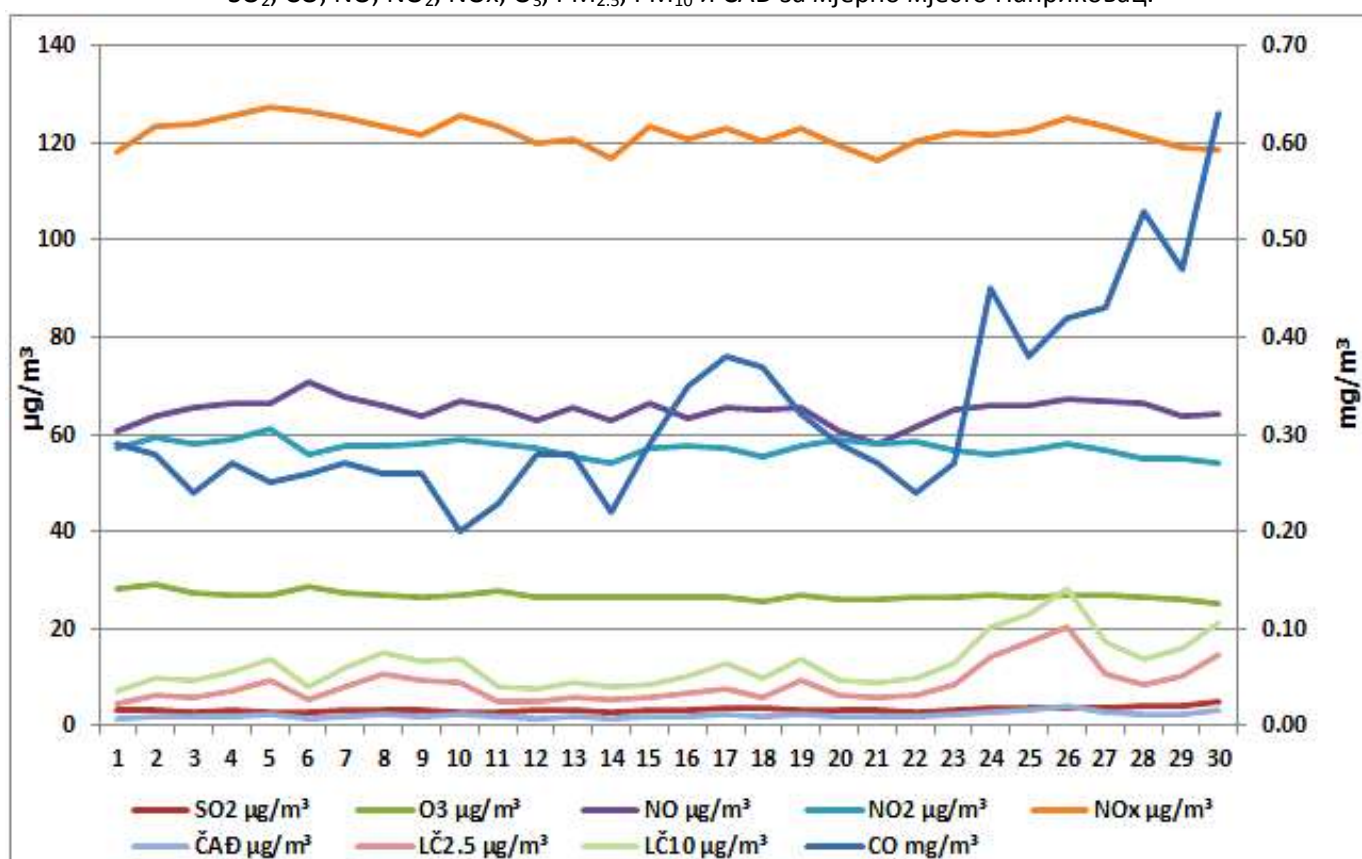
Дијаграм 2. Графички приказ просјечних имисијских дневних концентрација SO 2 ,CO, NO, NO 2 , NO x , O 3 , PM 2.5 , PM 10 и ЧАД за септембар 2025. у Бањој Луци (мјерно мјесто Паприковац)
