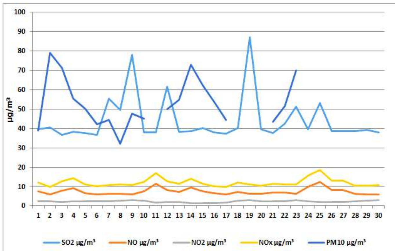
Дијаграм 8. Графички приказ просјечних имисијских дневних концентрација SO 2 , NO, NO 2 , Nox и PM 10 честица за септембар 2025. у Угљевику на мјерном мјесту-круг Т.Е.Угљевик.
