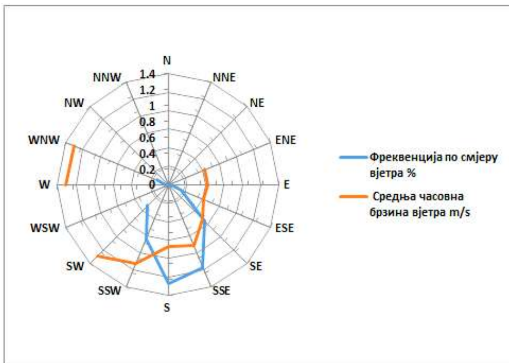
Слика 1. Приказ честине вјетра за септембар 2025. у Гацку (мјерном мјесту круг ОШ „Свети Сава“).
