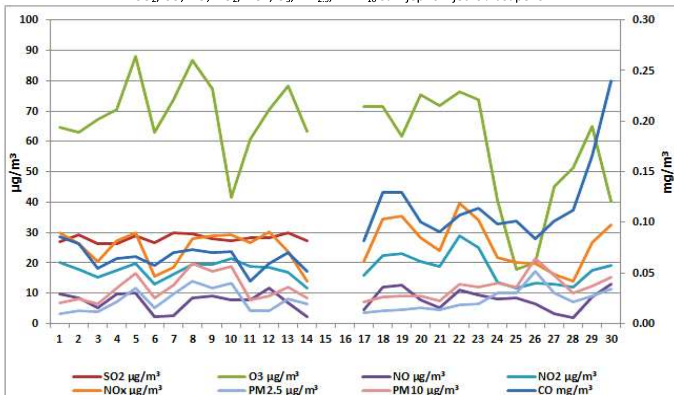
Дијаграм 1. Графички приказ просјечних имисијских дневних концентрација SO 2 , CO, NO, NO 2 , NO x , O 3 , PM 2.5 , и PM 10 за септембар 2025 у Бањој Луци (мјерно мјесто Лазарево).
