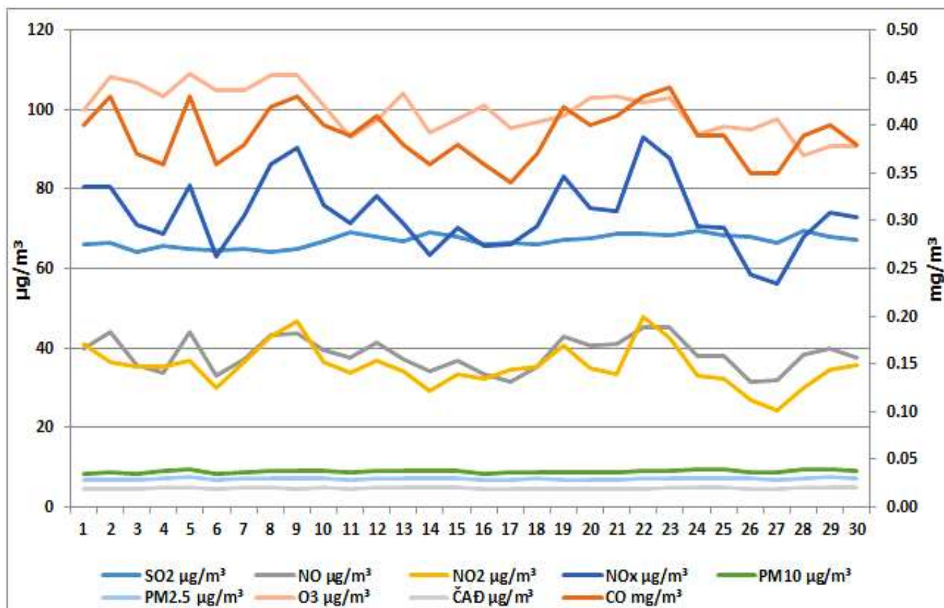
Дијаграм 6. Графички приказ просјечних имисијских дневних SO 2 , CO, NO, NO 2 , NO x , O 3 , ČАД, PM 2.5 и PM 10 за септембар 2025. у Бијељини (мјерно мјесто Центар града).
