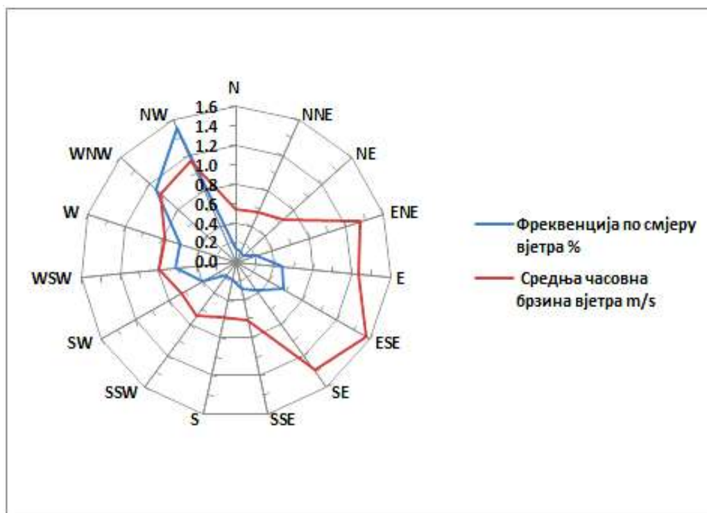
Слика 3. Приказ честине вјетра за септембар 2025. године у Броду (мјерно мјесто Рафинерија нафте Брод а.д.)
