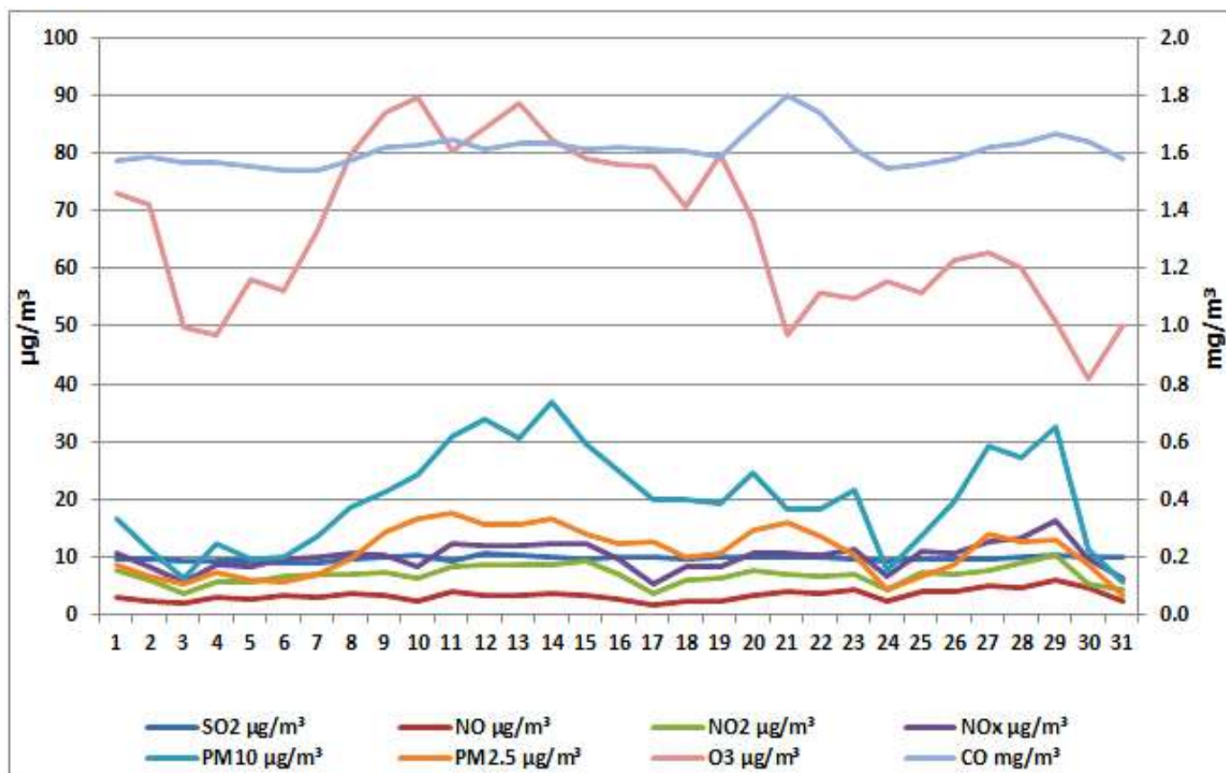
Дијаграм 2. Графички приказ просјечних имисијских дневних концентрација SO 2 , NO, NO 2 , NO x , PM 2.5 , PM 10 , CO и O 3 за август 2025. у Приједору (мјерно мјесто круг метеоролошке станице у Приједору)
