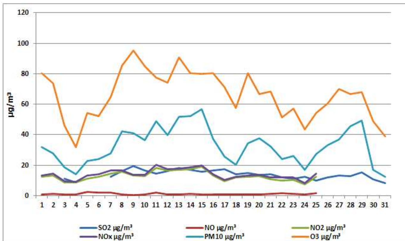
Дијаграм 9. Графички приказ просјечних имисијских дневних концентрација NO, NO 2 , NO x , PM 10 , O 3 и SO 2 за август 2025. у Добоју (мјерно мјесто круг метеоролошке станице у Добоју)
