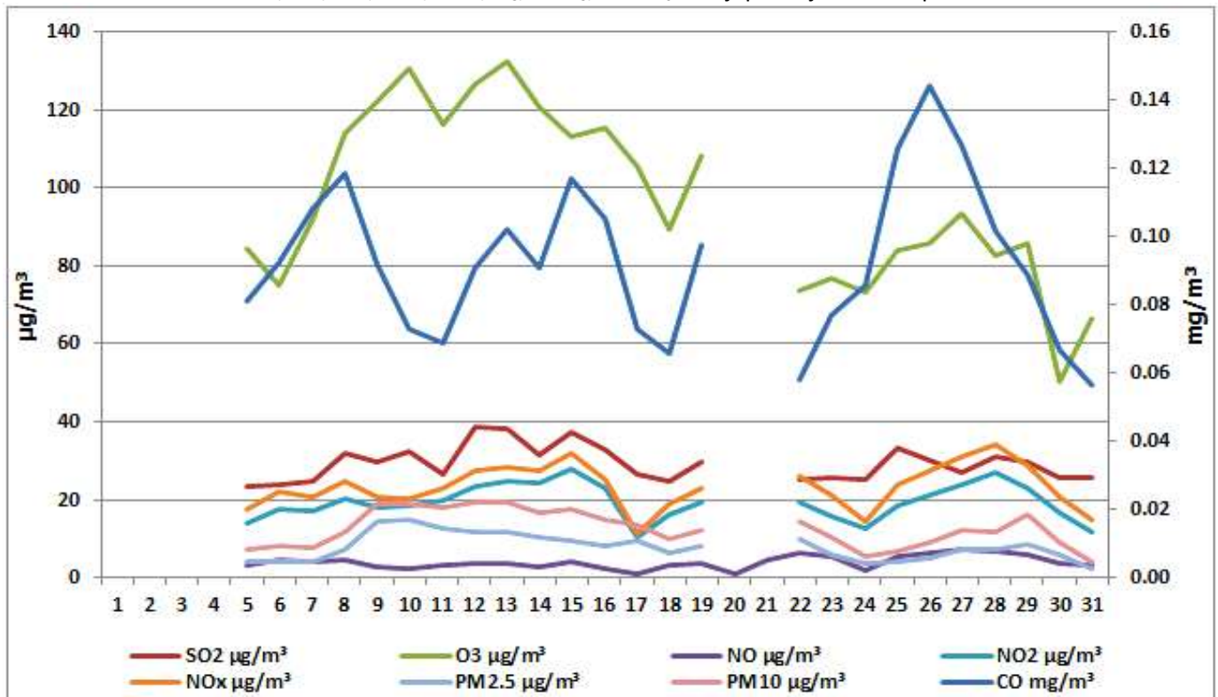
Дијаграм 1. Графички приказ просјечних имисијских дневних концентрација SO 2 , CO, NO, NO 2 , NO x , O 3 , PM 2.5 , и PM 10 за август 2025 у Бањој Луци (мјерно мјесто Лазарево).
