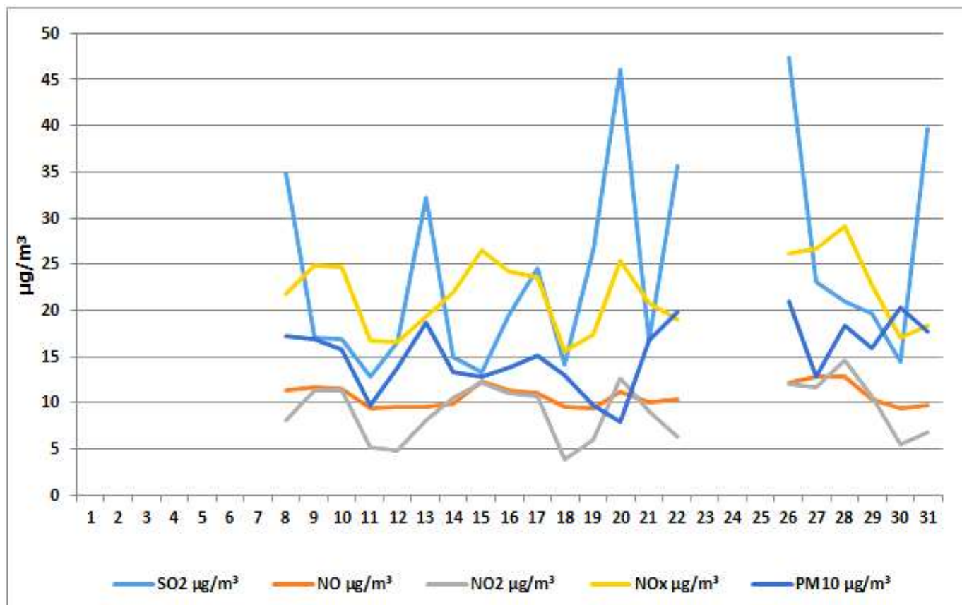
Дијаграм 5. Графички приказ просјечних имисијских дневних концентрација \text{SO}_2 , \text{PM}_{10} , \text{NO} , \text{NO}_2 и \text{NO}_x за август 2025. у Гацку (мјерном мјесту круг ОШ „Свети Сава“).
