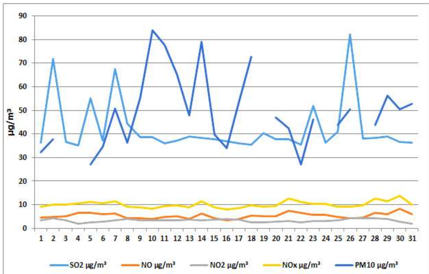
Дијаграм 6. Графички приказ просјечних имисијских дневних концентрација \text{SO}_2 , \text{NO} , \text{NO}_2 , \text{NO}_x и \text{PM}_{10} честица за август 2025. у Угљевику на мјерном мјесту-круг Т.Е.Угљевик.
