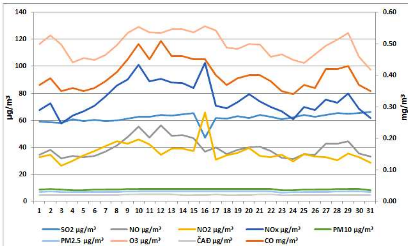
Дијаграм 3. Графички приказ просјечних имисијских дневних SO 2 , CO, NO, NO 2 , NO x , O 3 , ČАД, PM 2.5 и PM 10 за август 2025. у Бијељини (мјерно мјесто Центар града).
