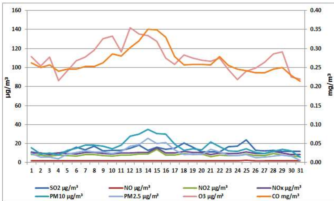
Дијаграм 8. Графички приказ просјечних имисијских дневних концентрација SO 2 , NO, NO 2 , NO x , CO, PM 10 , O 3 и PM 2.5 честица за август 2025. у Требињу (мјерно мјесто круг метеоролошке станице у Требињу)
