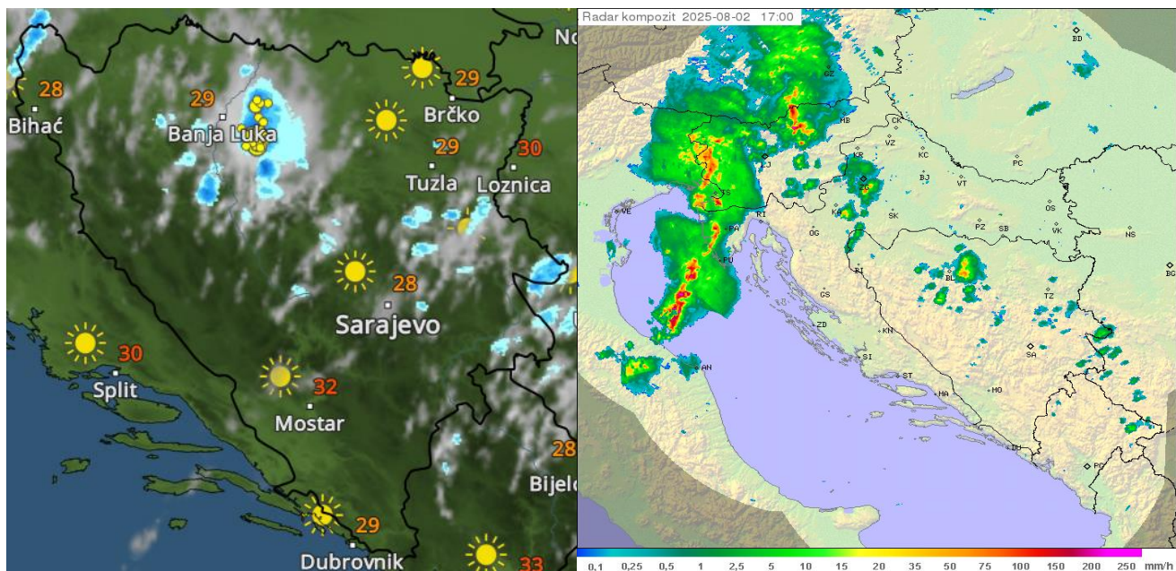
Сателитска и радарска слика 02.08. у 17 часова (Извор wetteronline.de и DHMZ)
