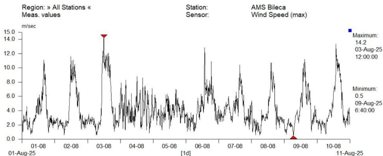
Удари вјетра у периоду 01.-11.08.2025. за АМС Билећа (извор: РХМЗРС)
