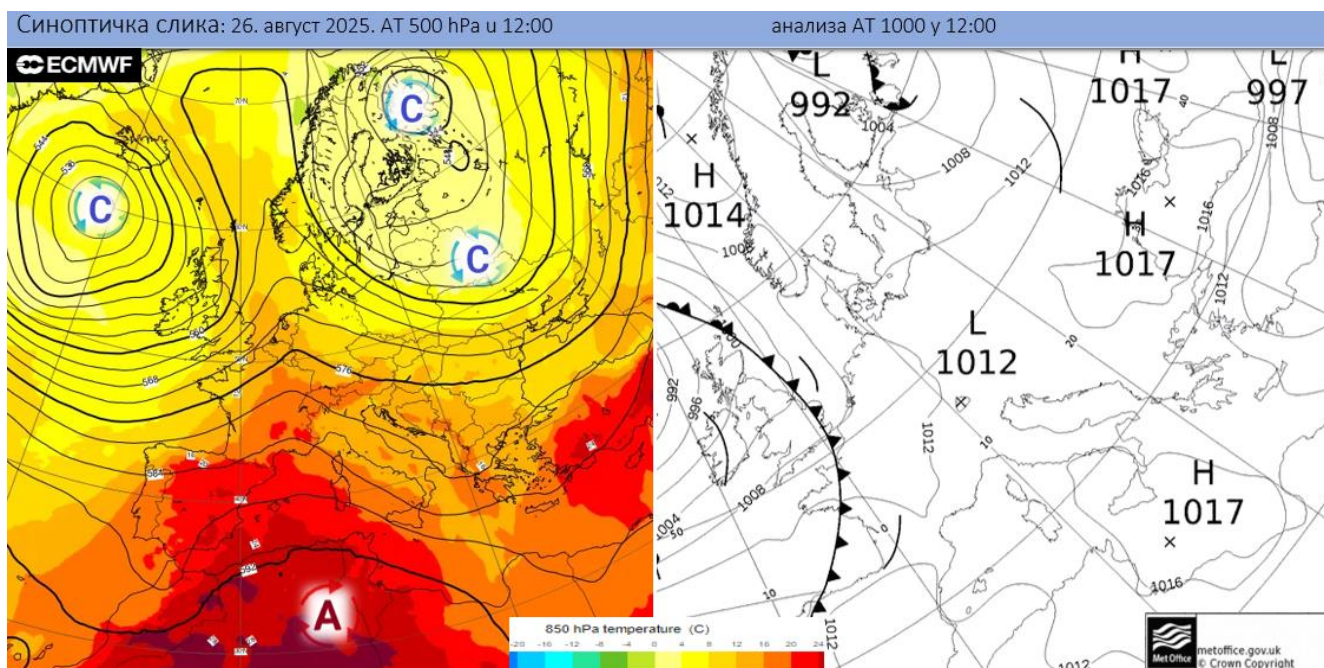
Синоптичка ситуација 26.08. у подне (извор: ECMWF и wetter3.de)
