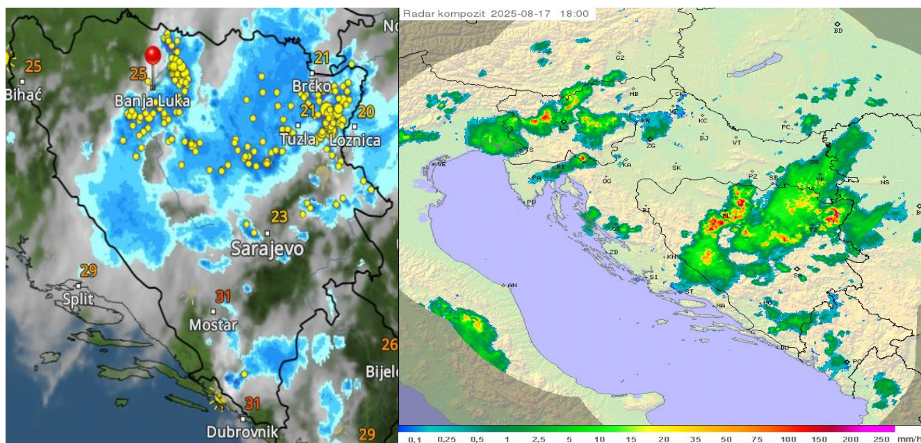
Сателитска и радарска слика 17.08. у 18 часова (Извор wetteronline.de и DHMZ)
