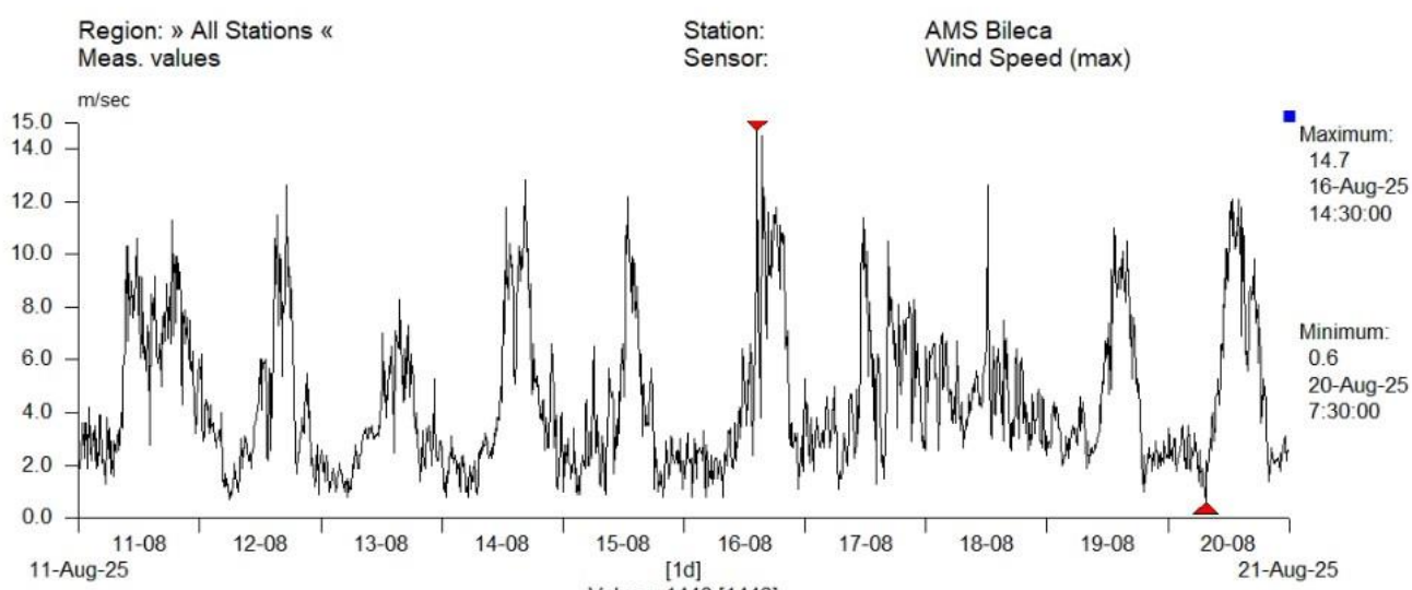
Удари вјетра у периоду 11.-21.08.2025. за АМС Билећа (извор: РХМЗРС)
