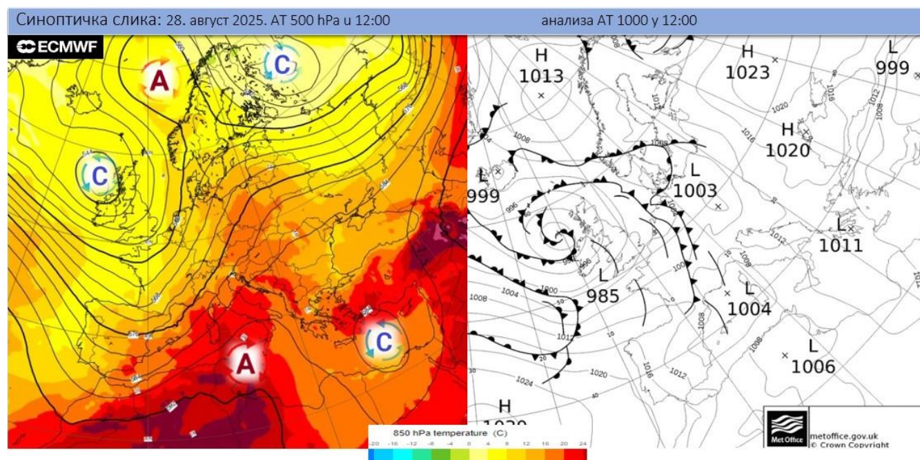
Синоптичка ситуација 28.08. у подне (извор: ECMWF и wetter3.de)
