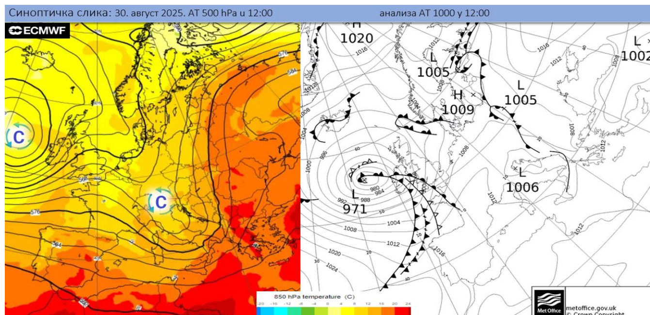
Синоптичка ситуација 30.08. у подне (извор: ECMWF и wetter3.de)
