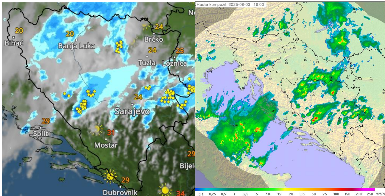
Сателитска и радарска слика 03.08. у 16 часова (Извор: wetteronline.de и DHMZ)
