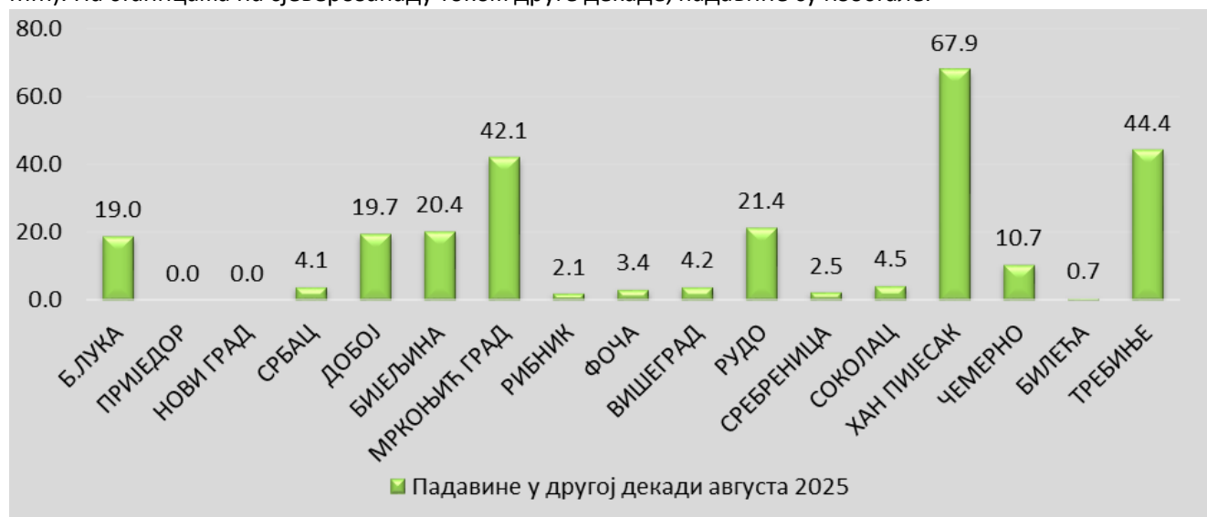
Падавине у другој декади августа 2025. (РХМЗРС)
