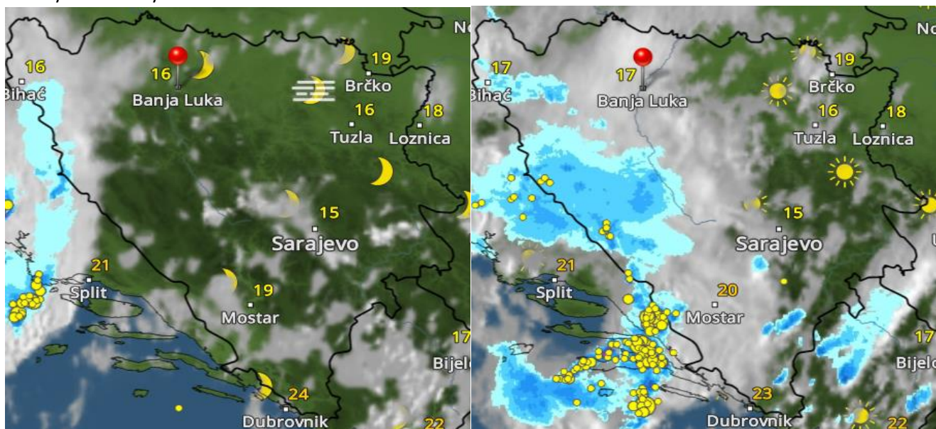
Сателитске слике у 04 и 07 часова 22.08. (Извор: wetteronline.de)
