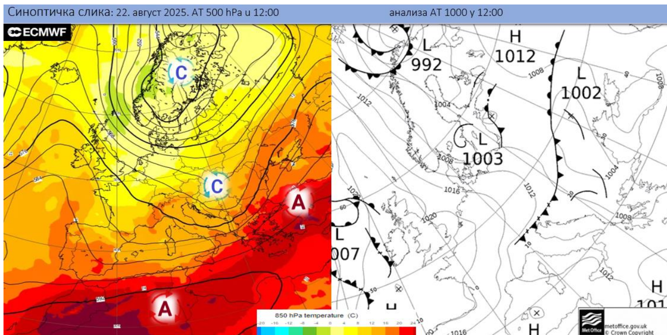
Синоптичка ситуација 22.08. у подне (извор: ECMWF и wetter3.de)
