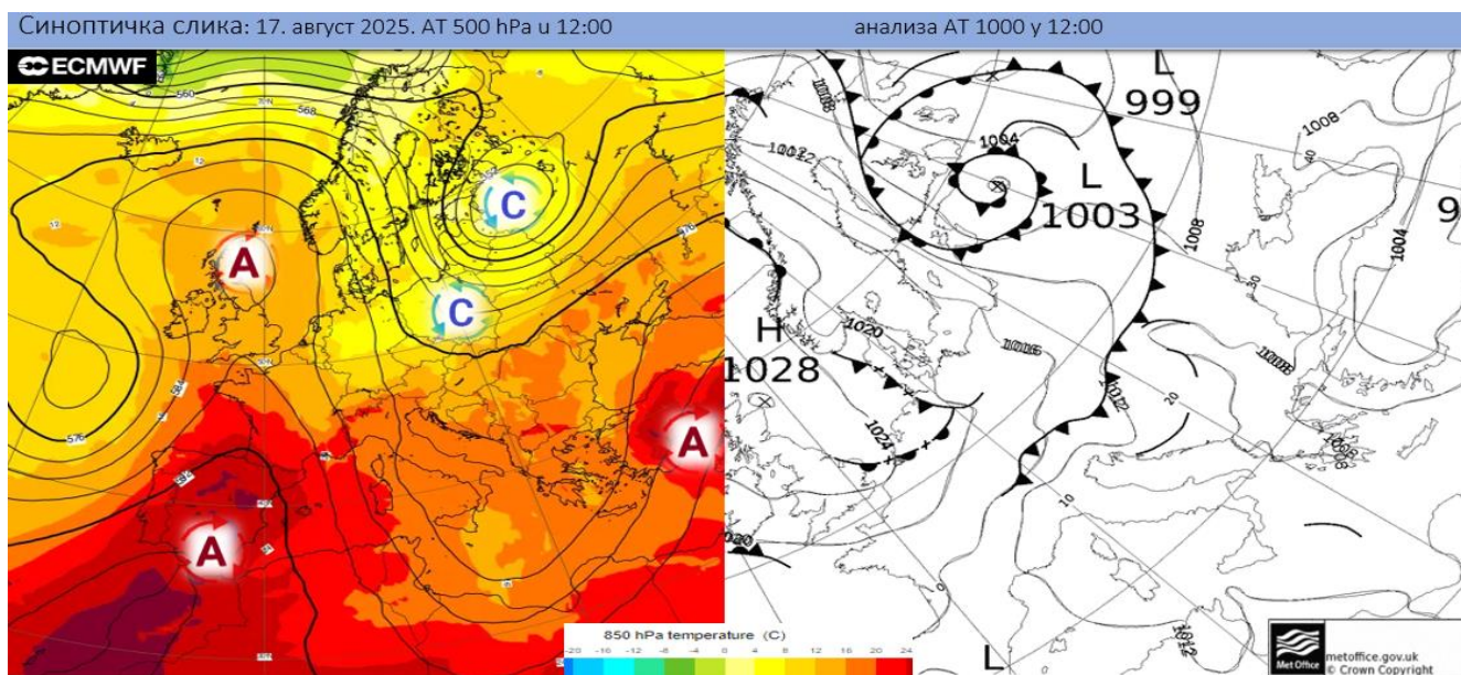
Синоптичка ситуација 17.08. у подне (извор: ECMWF и wetter3.de)
