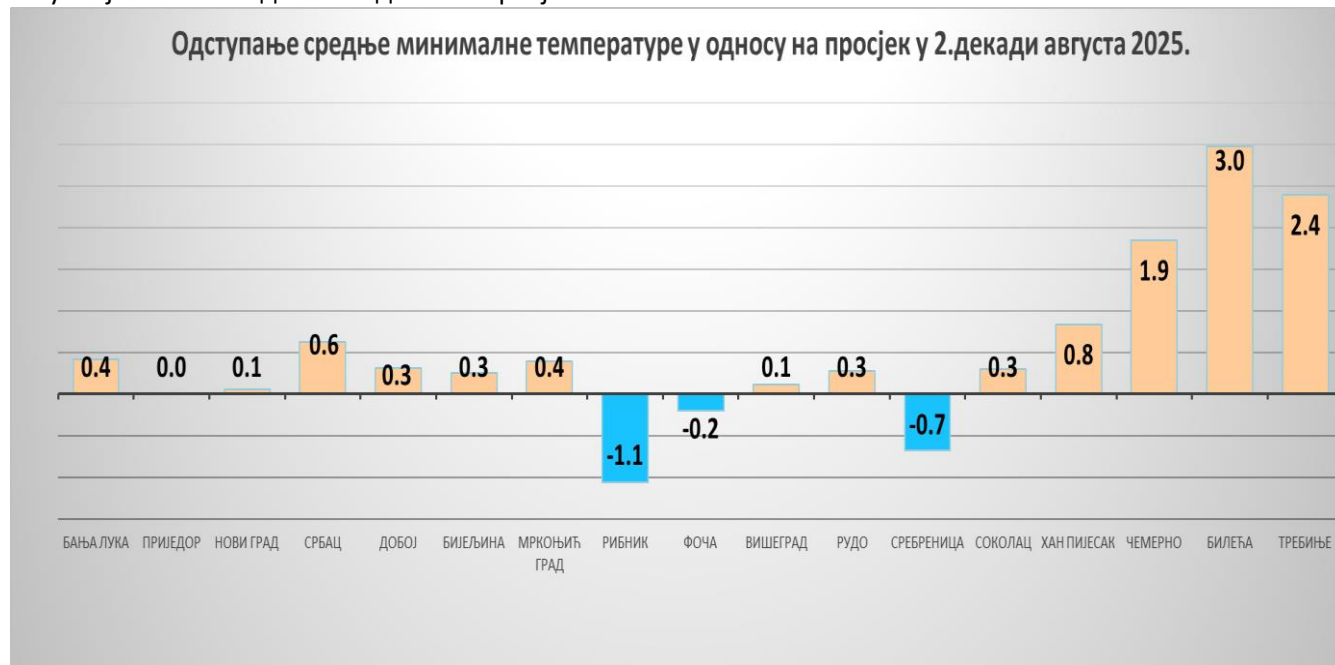
Одступање средње минималне температура ваздуха у другој декади августа у односу на вишегодишњи просјек (РХМЗРС)
